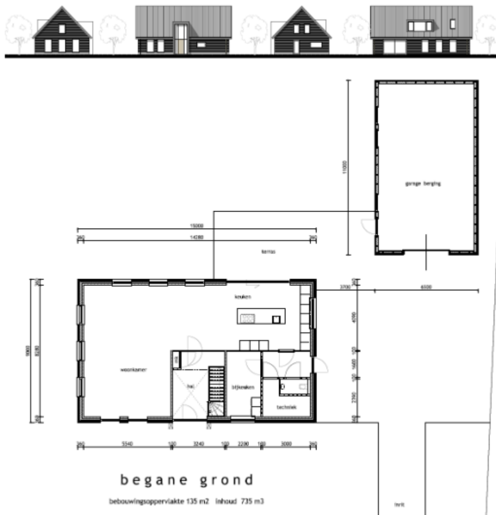
Figuur 3 Plattegronden beoogde woning
