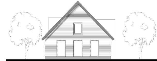
zijgevel
