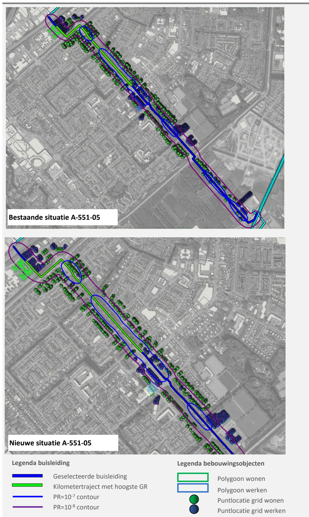
Figuur 6.1: Ingevoerde omgevingsobjecten in CAROLA en PR-contouren en hoogste GR-tracé leiding A-551-05
