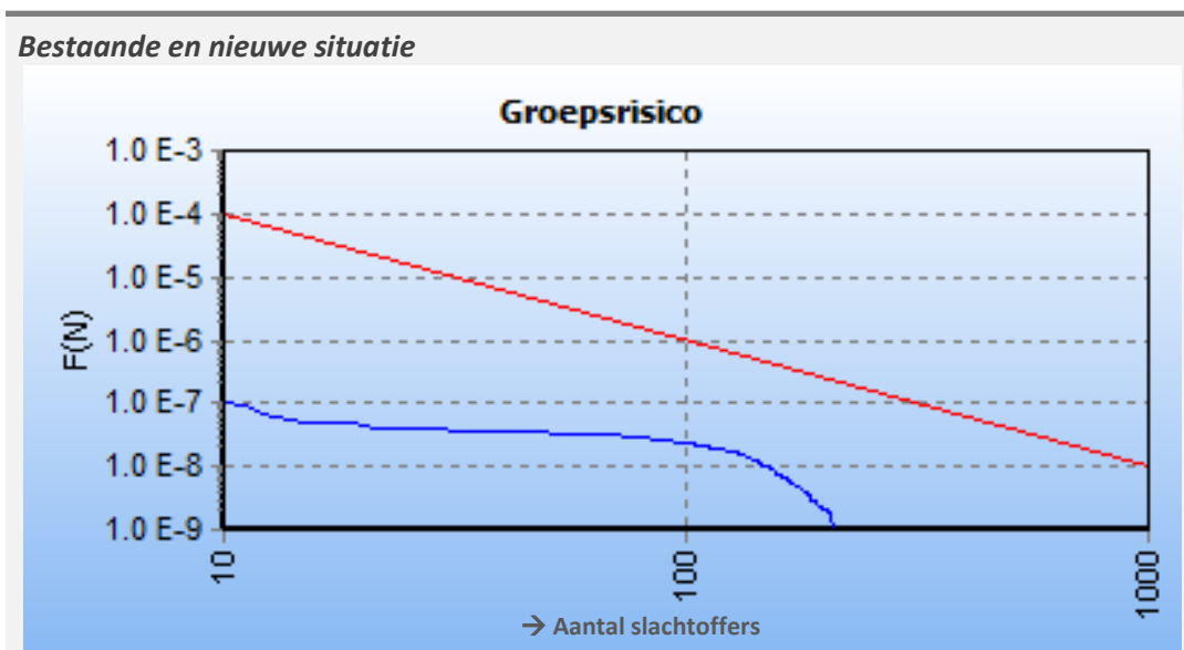
Figuur 6.3 FN curve voor buisleiding A-551-05 van Gasunie voor de kilometer tussen stationing 1760.00 en 2760.00 (bestaande en nieuwe situatie)
