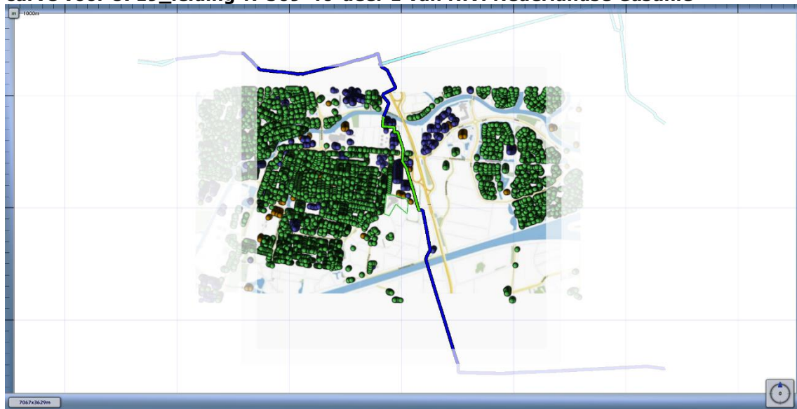
Figuur 4.2 Kilometer leiding behorende bij de maximale overschrijding van de FN-curve voor 8719_leiding-N-509-40-deel-1 van N.V. Nederlandse Gasunie
