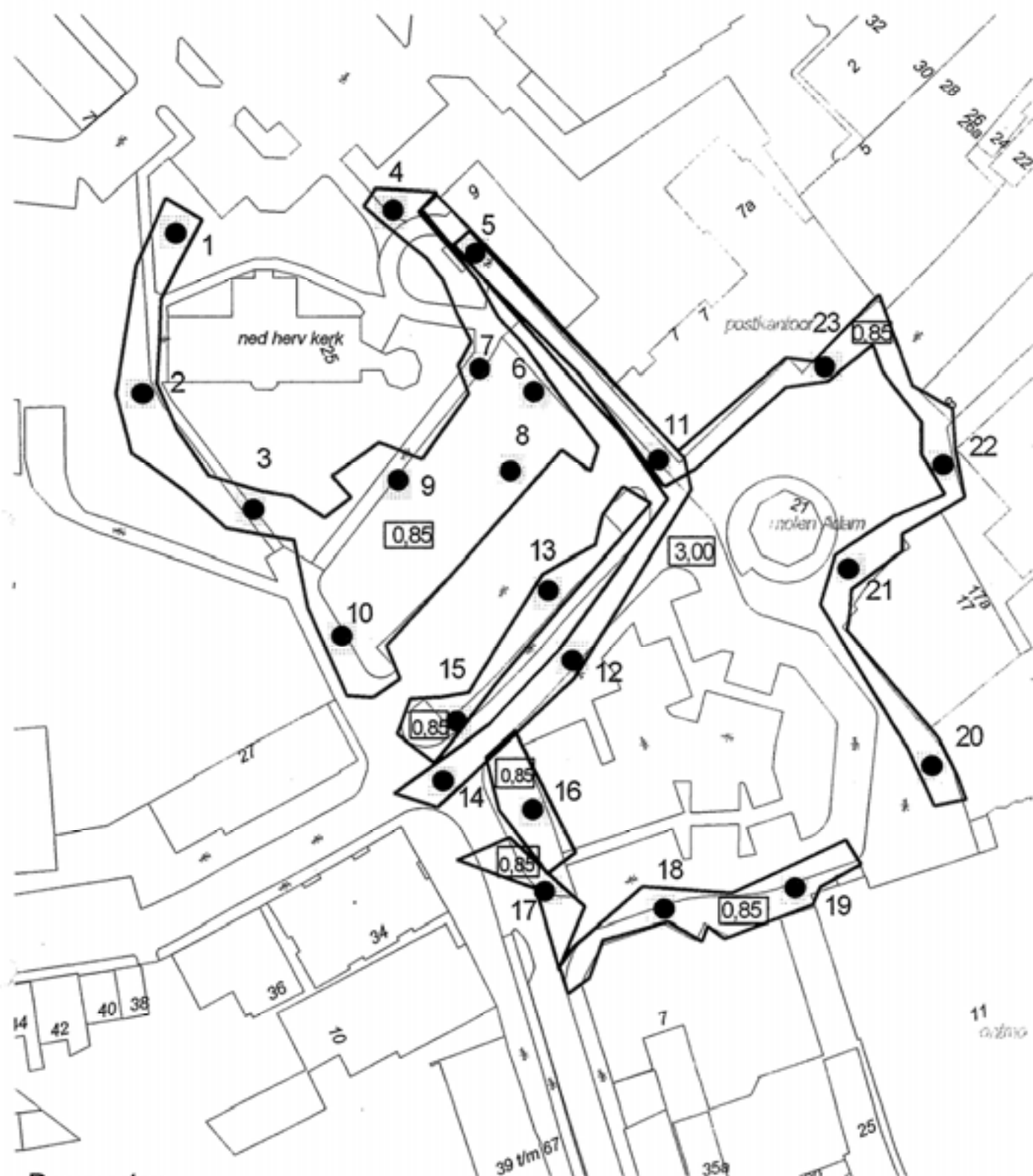
Bijlage 2: Terreinoverzicht en ligging van de boorpunten
