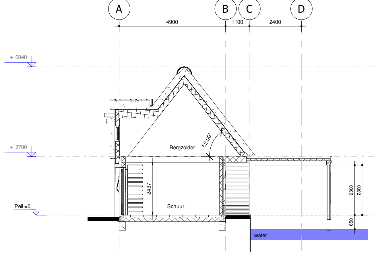
Doorsnede - B -
