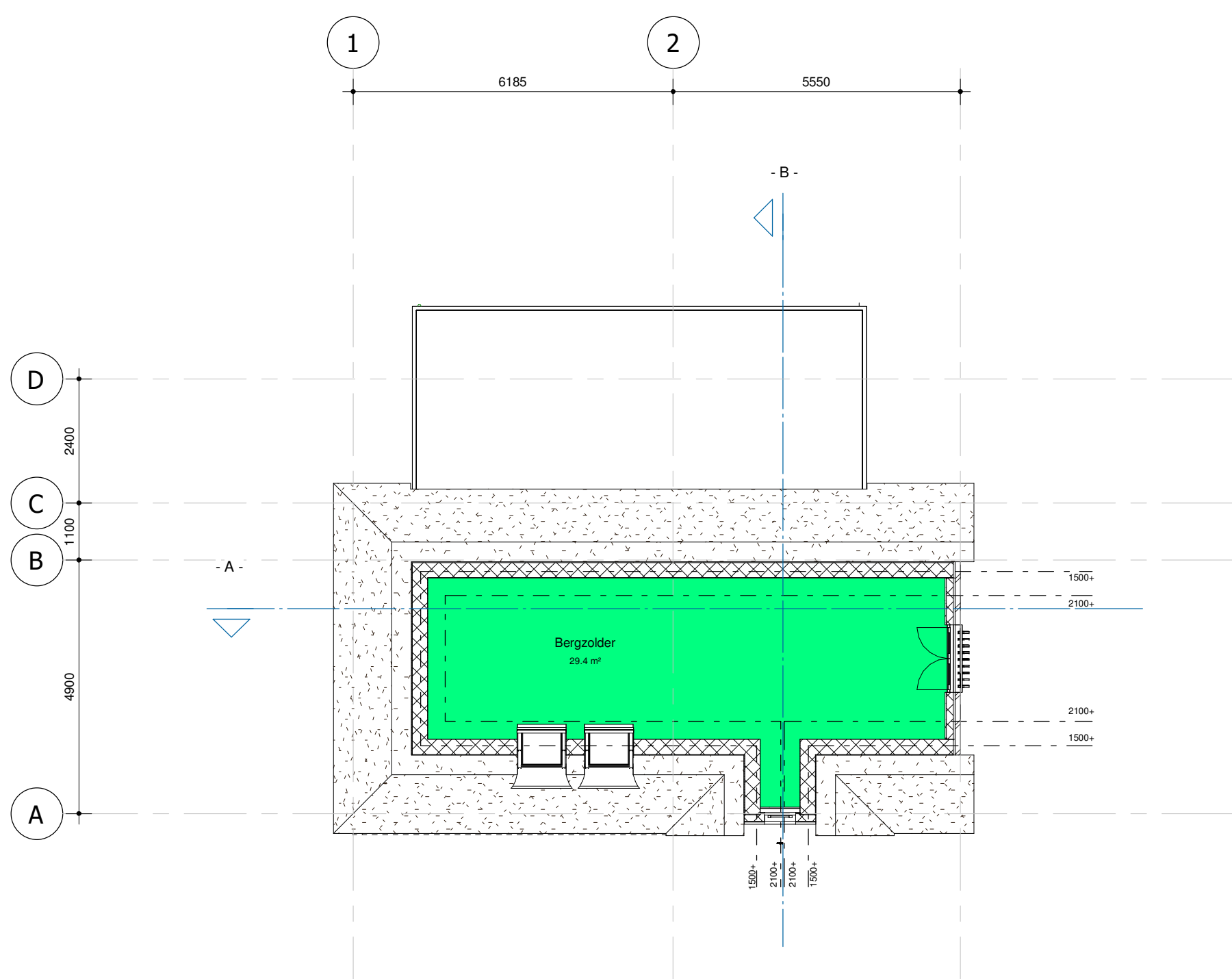
Eerste verdieping
