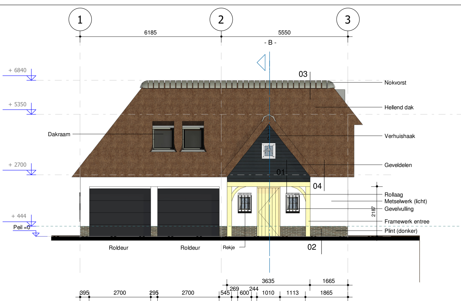
Rechter zijgevel
