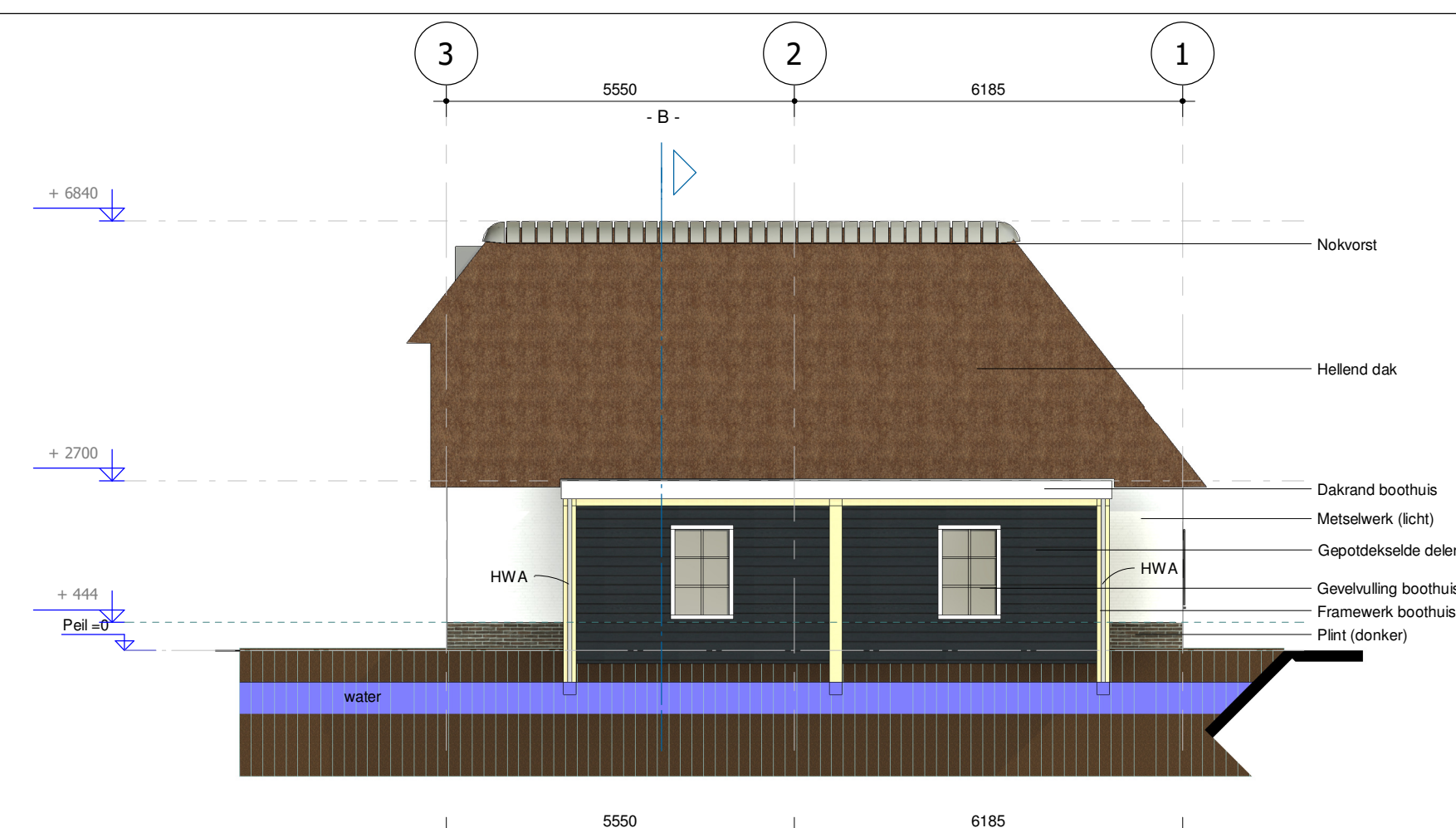
Linker zijgevel
