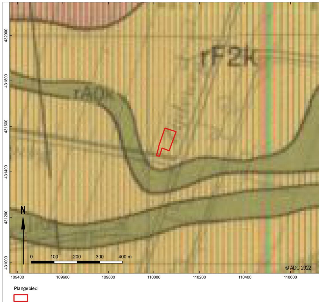
Afb. 4. Het plangebied op de geologische kaart 1982 (Rijksgeologische Dienst)
