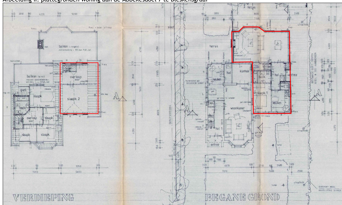
Afbeelding II: plattegronden woning aan de Abbekesdoel 7 te Bleskensgraaf
