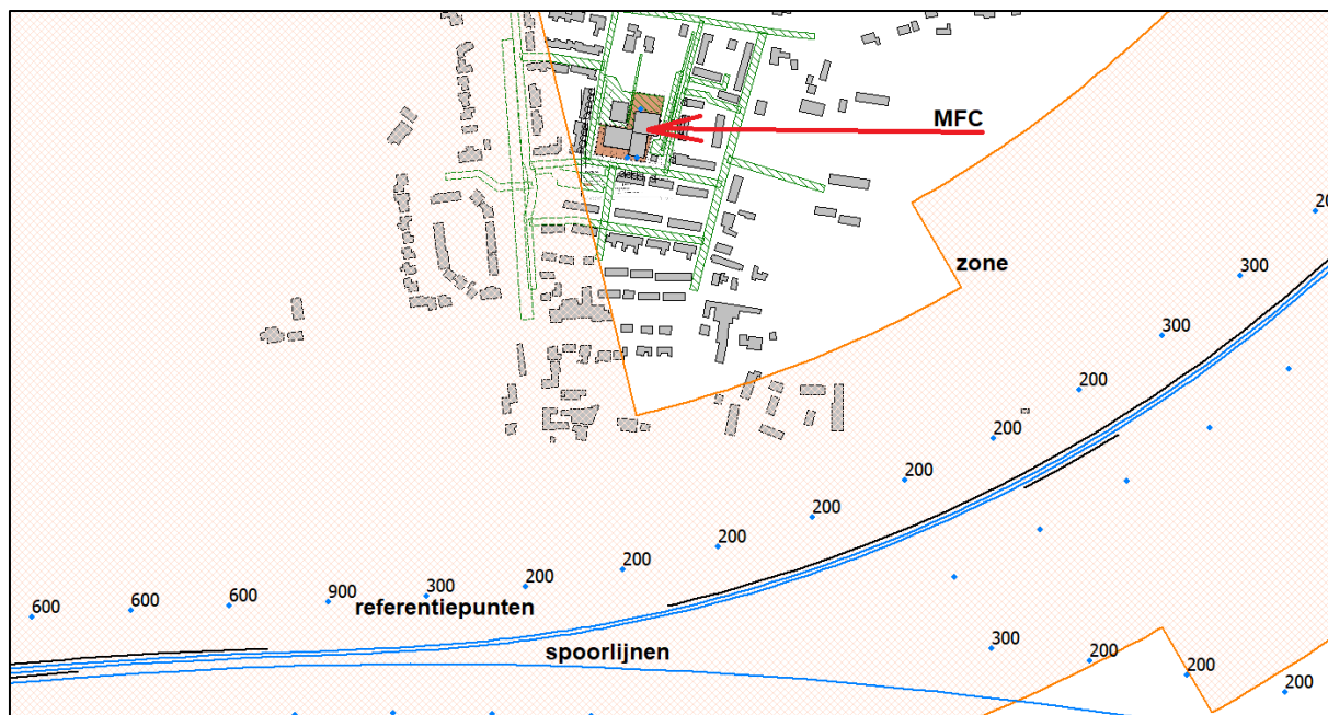
Figuur 1 Omvang zone railverkeerslawaaï
