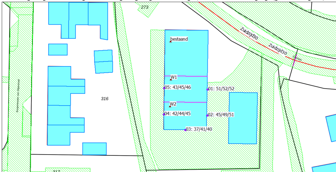
Afbeelding VII: gecumuleerde geluidbelasting ten gevolge van alle wegen, excl. aftrek art. 110g Wgh (gevelmaatregelen)
