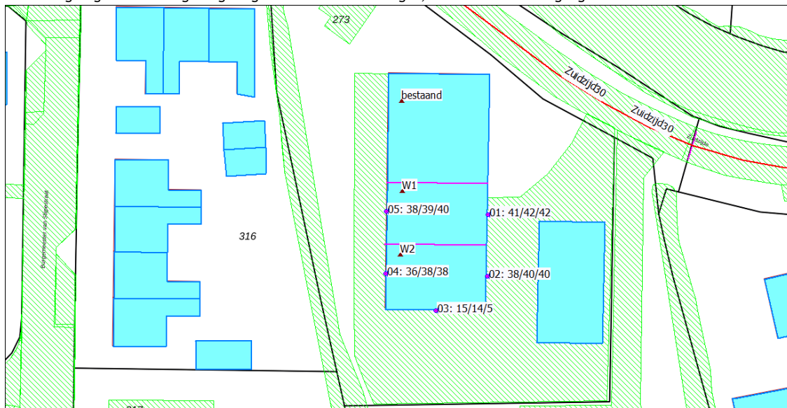
Afbeelding V: geluidbelasting ten gevolge van alle 30 km/h wegen, incl. aftrek art. 110g Wgh
