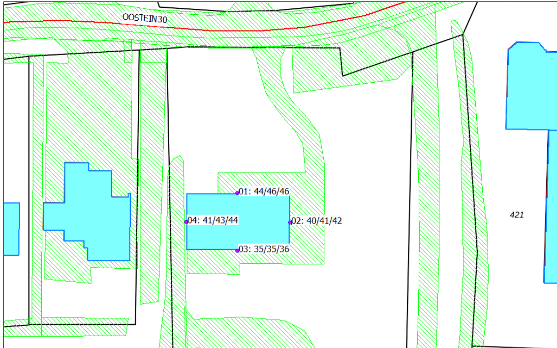
Afbeelding VI: gecumuleerde geluidbelasting ten gevolge van alle wegen, excl. aftrek art. 110g Wgh (gevelmaatregelen)
