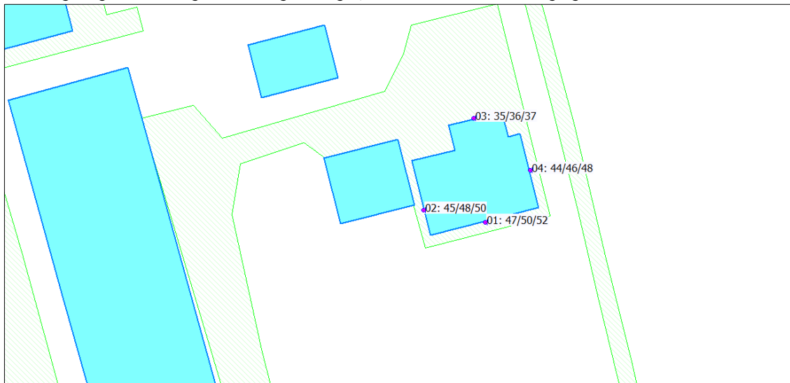
Afbeelding VII: gecumuleerde geluidbelasting alle wegen, incl. aftrek conform art. 110g Wgh
