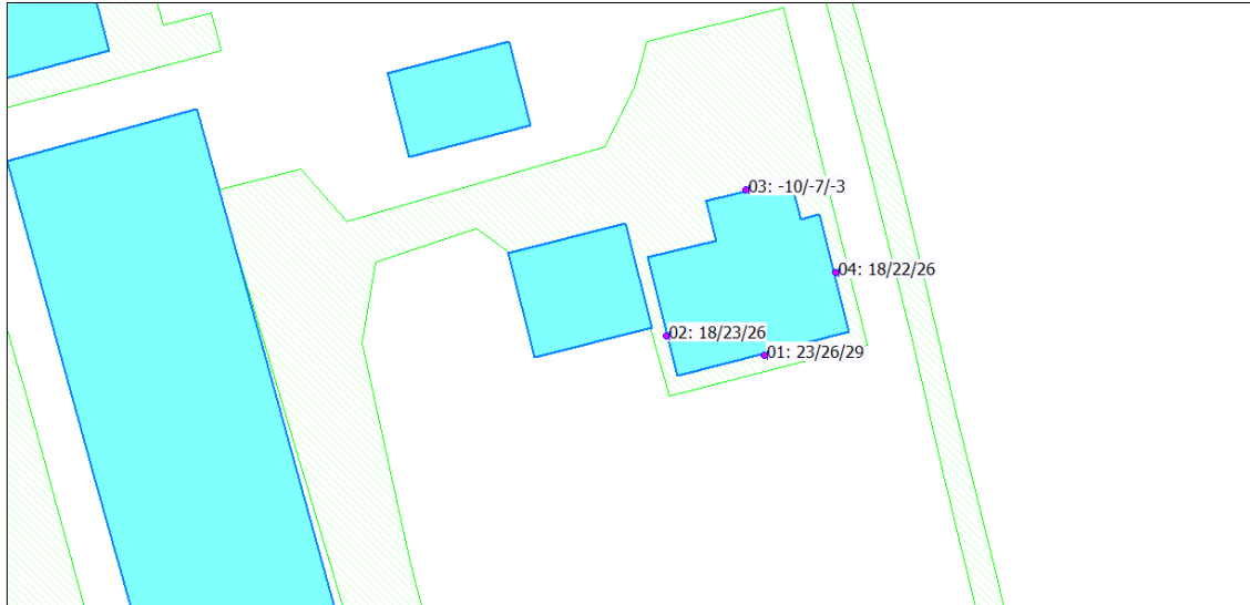
Afbeelding VI: geluidbelasting Grotewaard, incl. aftrek conform art. 110g Wgh
