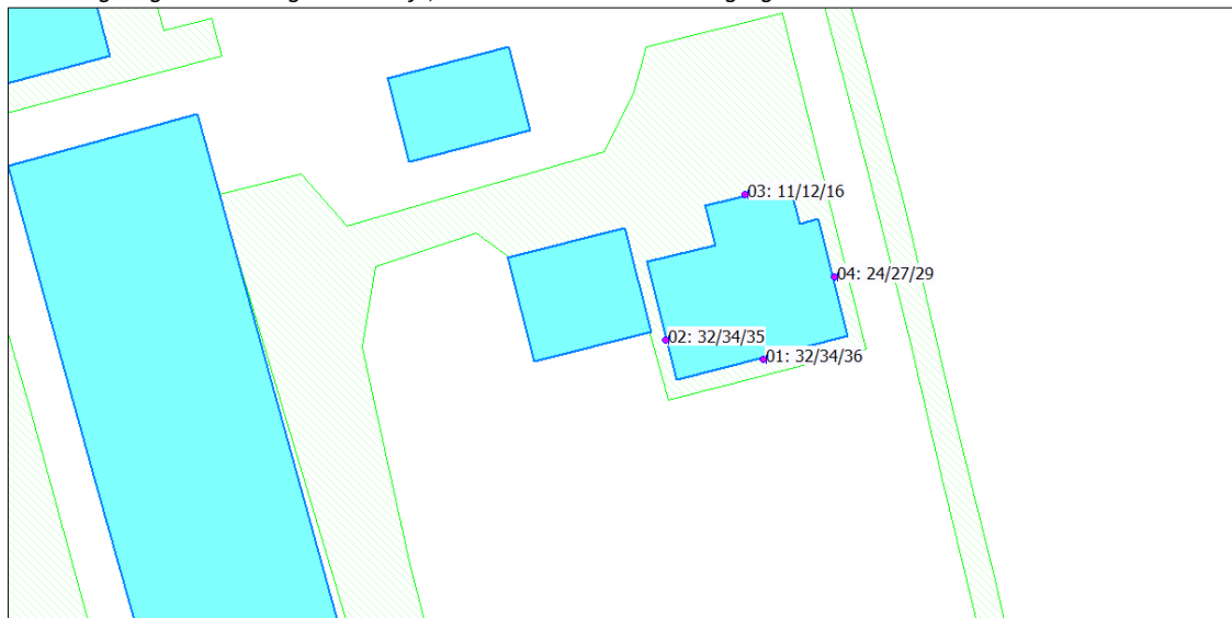
Afbeelding IV: geluidbelasting Nieuwendijk, incl. aftrek conform art. 110g Wgh
