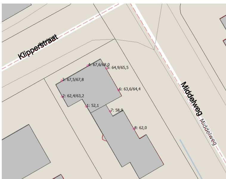
f4 Overzicht gecumuleerde geluidbelasting per rekenpunt [dB(A)] in de huidige situatie
