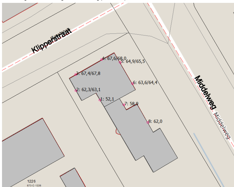
f5 Overzicht gecumuleerde geluidbelasting per rekenpunt inclusief aftrek [dB(A)] in de nieuwe situatie
