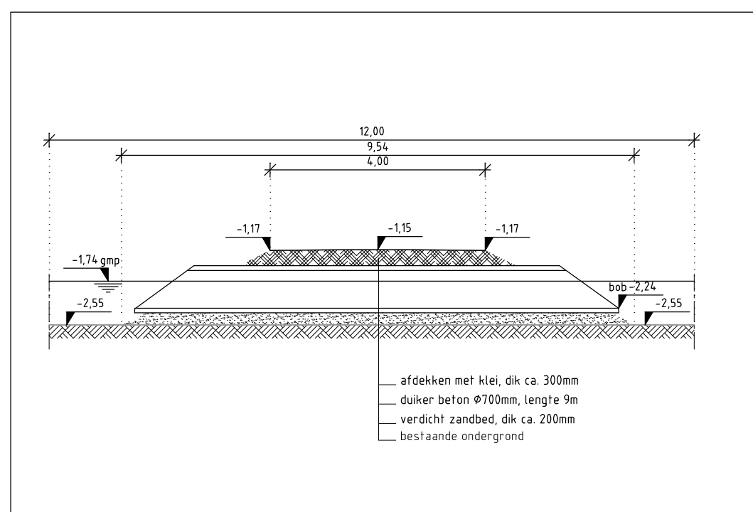
Profiel A langspandiel diiker
