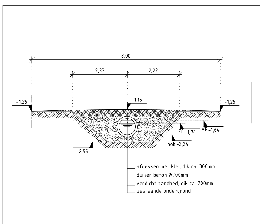
Profiel B dwarsprofiel diiker
