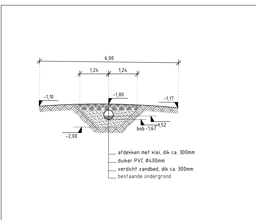
Profiel E dwarsprofiel diiker
