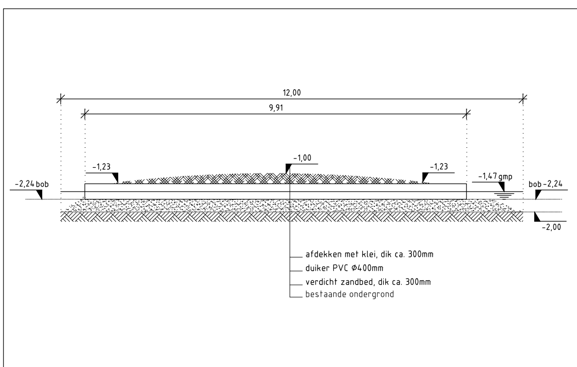
Profiel D langspandiel diiker
