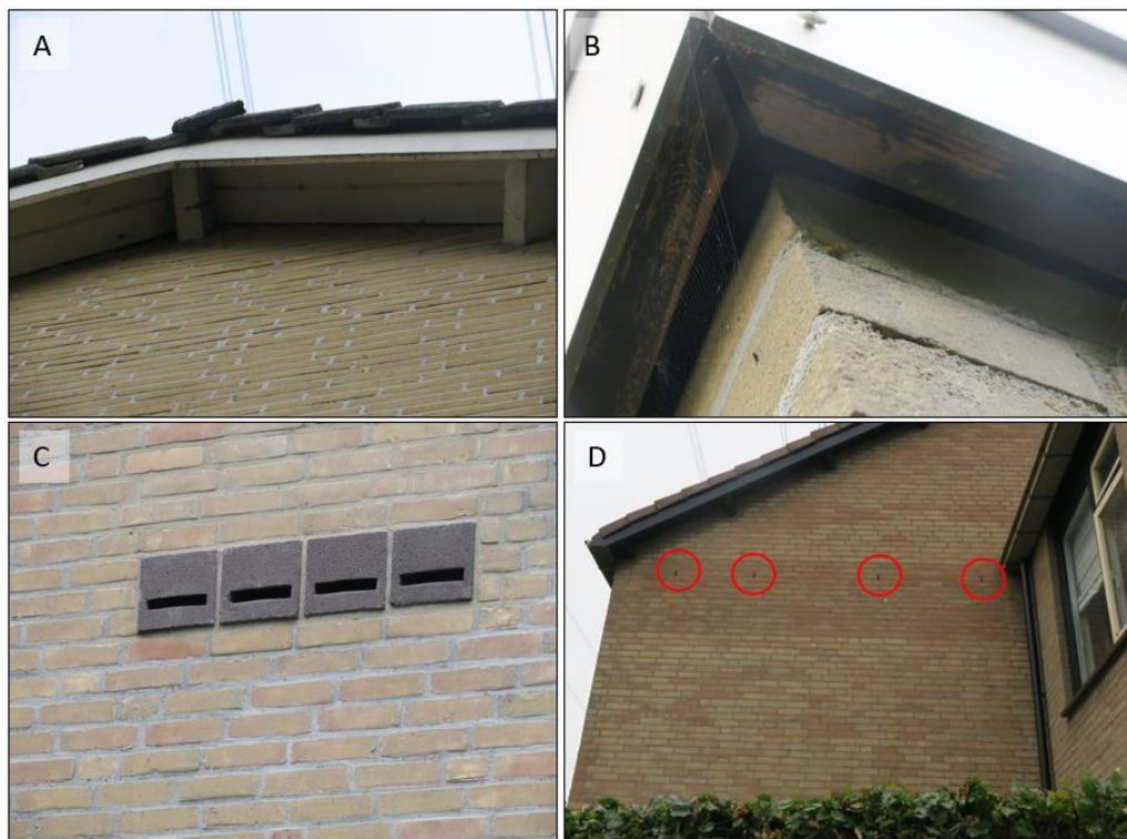
Figuur 5 Visuele representatie van geschikte invliegopeningen voor vleermuizen. (A) kierende kantpannen, (B) kier onder boeiboord van schuur, (C) vleermuis inbouwkasten, (D) open stootvoegen.
