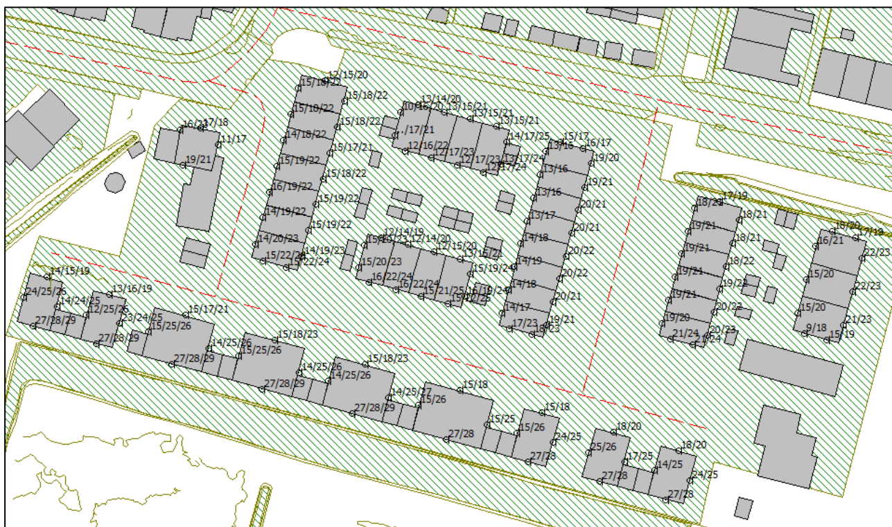
Figuur 4.2: Overzicht rekenmodel inclusief rekenresultaten Grotewaard
