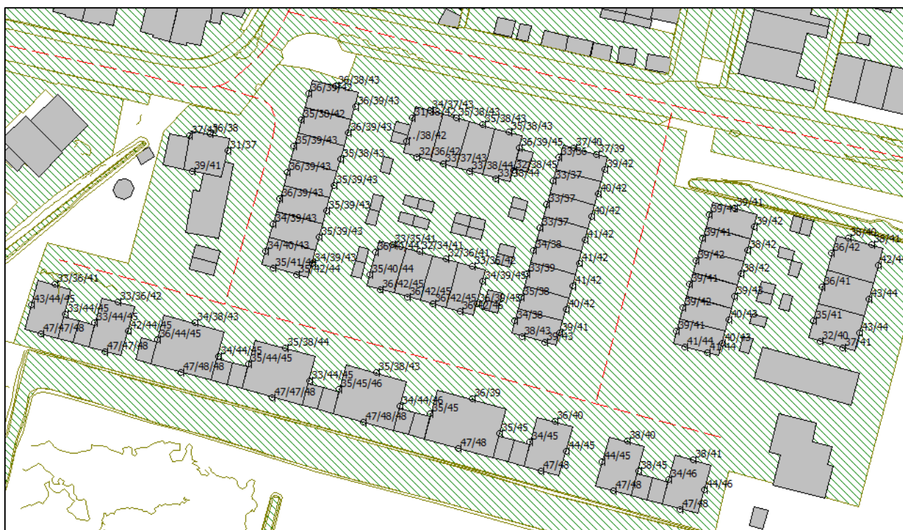
Figuur 4.3: Overzicht rekenmodel inclusief rekenresultaten N214
