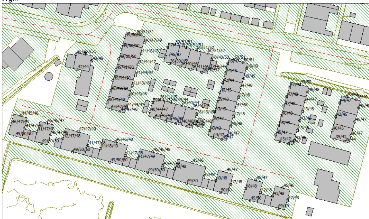
Figuur 4.4: Overzicht rekenmodel inclusief rekenresultaten wegen cumulatief
