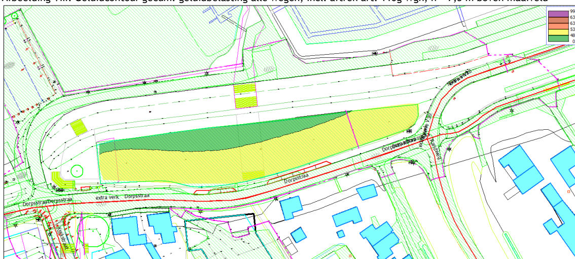
Afbeelding VIII: Geluidcontour gecum. geluidbelasting alle wegen, incl. aftrek art. 110g Wgh, h = 7,5 m boven maaiveld
