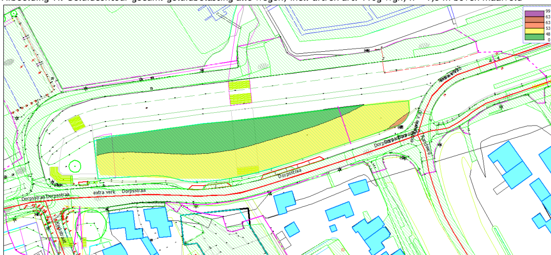
Afbeelding VI: Geluidcontour gecum. geluidbelasting alle wegen, incl. aftrek art. 110g Wgh, h = 1,5 m boven maaiveld
