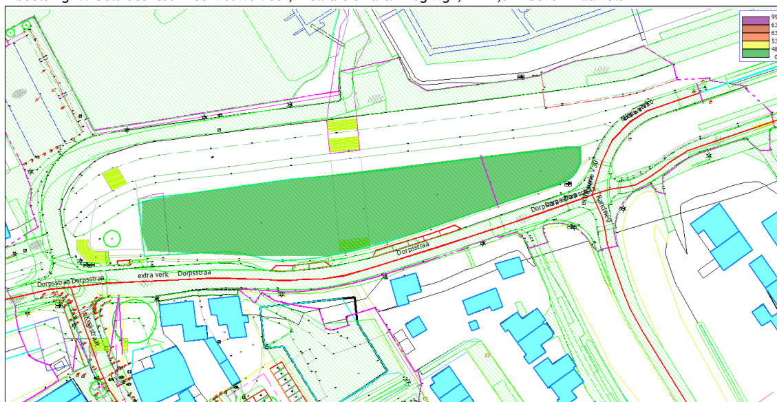
Afbeelding IV: Geluidcontour het Nieuwe Veer, incl. aftrek art. 110g Wgh, h = 4,5 m boven maaiveld
