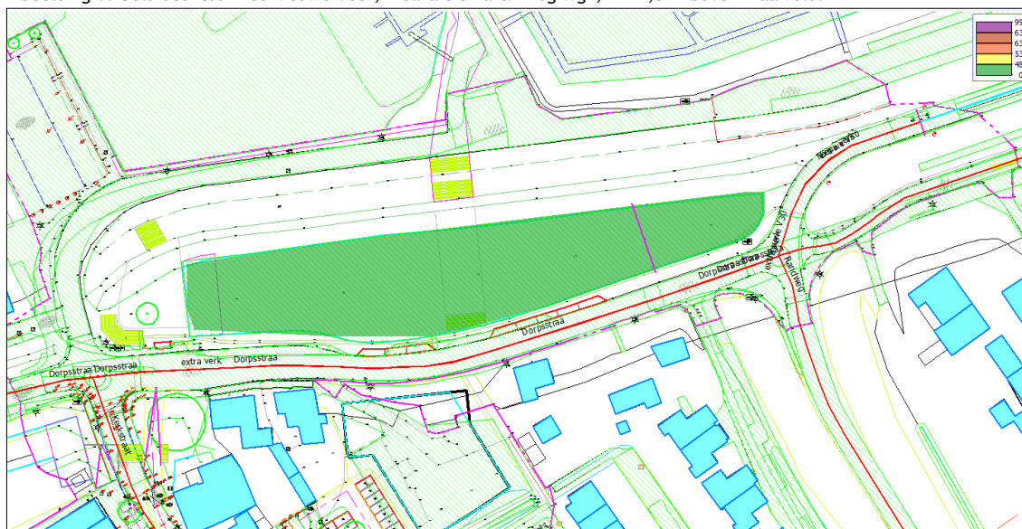
Afbeelding V: Geluidcontour het Nieuwe Veer, incl. aftrek art. 110g Wgh, h = 7,5 m boven maaiveld.
