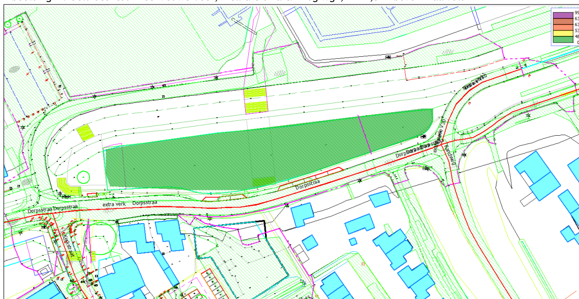
Afbeelding III: Geluidcontour het Nieuwe Veer, incl. aftrek art. 110g Wgh, h = 1,5 m boven maaiveld
