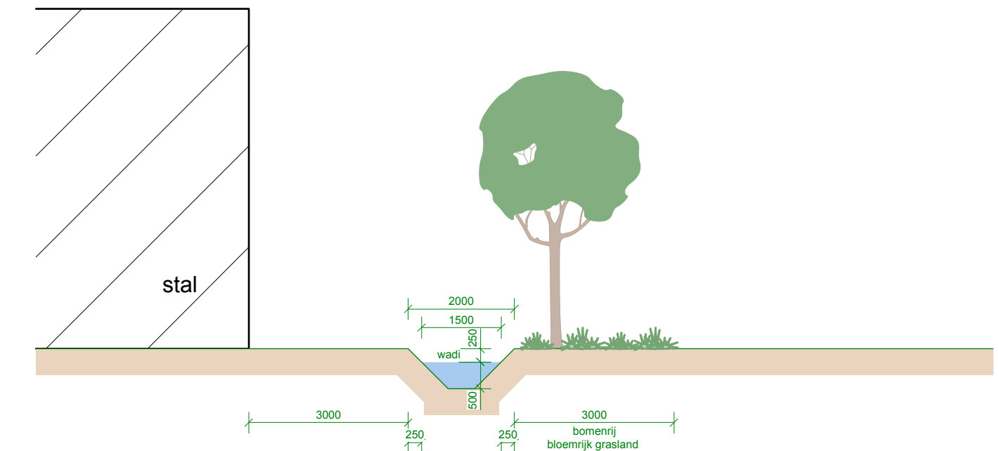
Doorsnede A schaal 1 : 100
