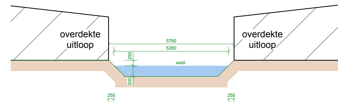
Doorsnede B schaal 1 : 100
