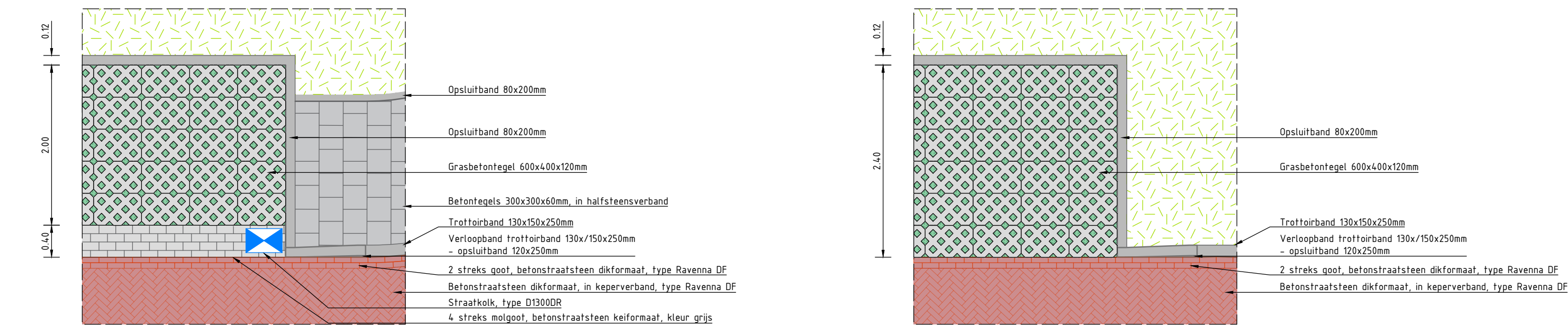
Detail 1 (parkeerstrook met molgoot) SCHAAL 1 : 50
