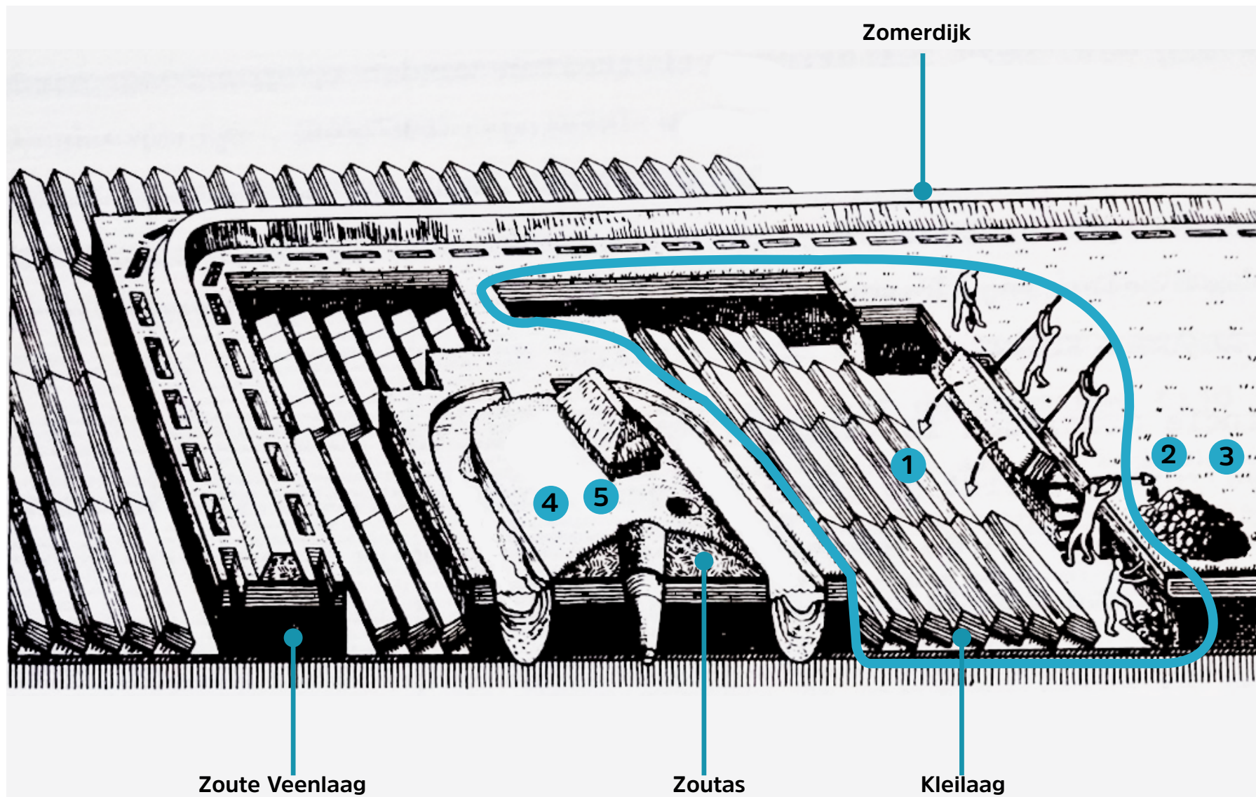
Afb.3.18 Schematische weergave van het zoutwinningsproces en het aangraven van de zoute veenlagen, naar Bantelmann 1966.
