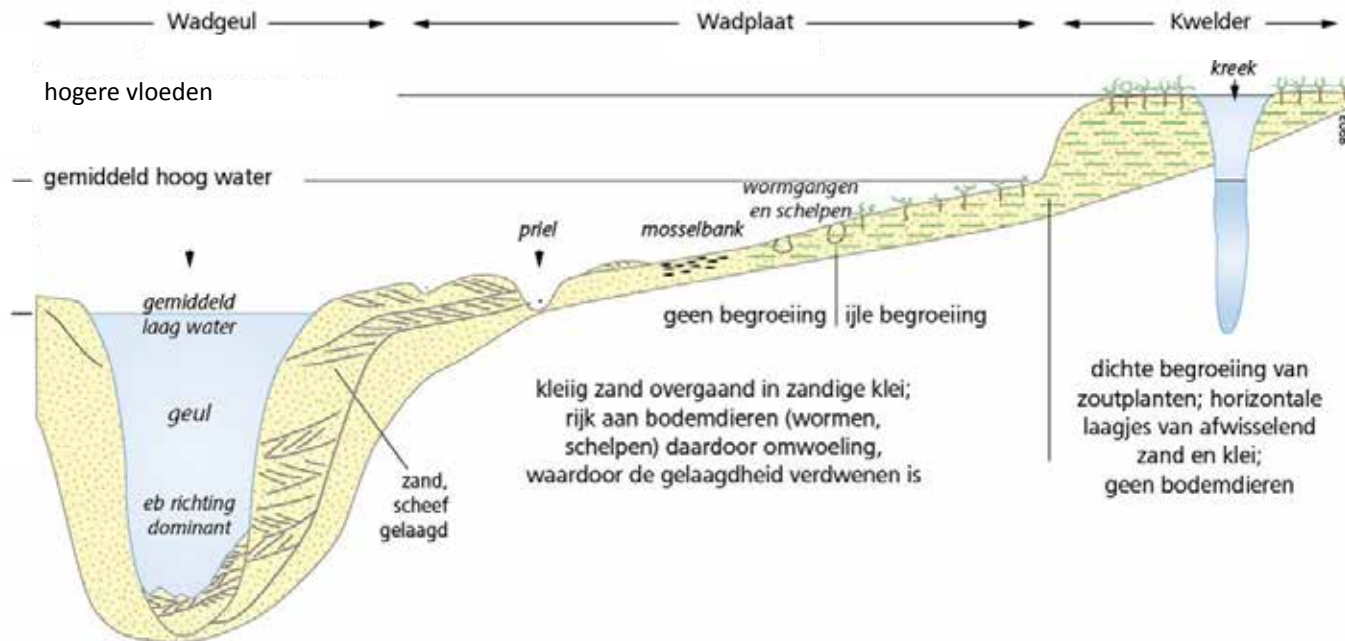
Afb.2.08 Wadgeul, zone met wadden en slikken en een kwelder afgezet tegen de getijdenwerking. Bovenop de kwelder kon zich een kwelderwal vormen die alleen bij hogere vloeden overstroomde.
