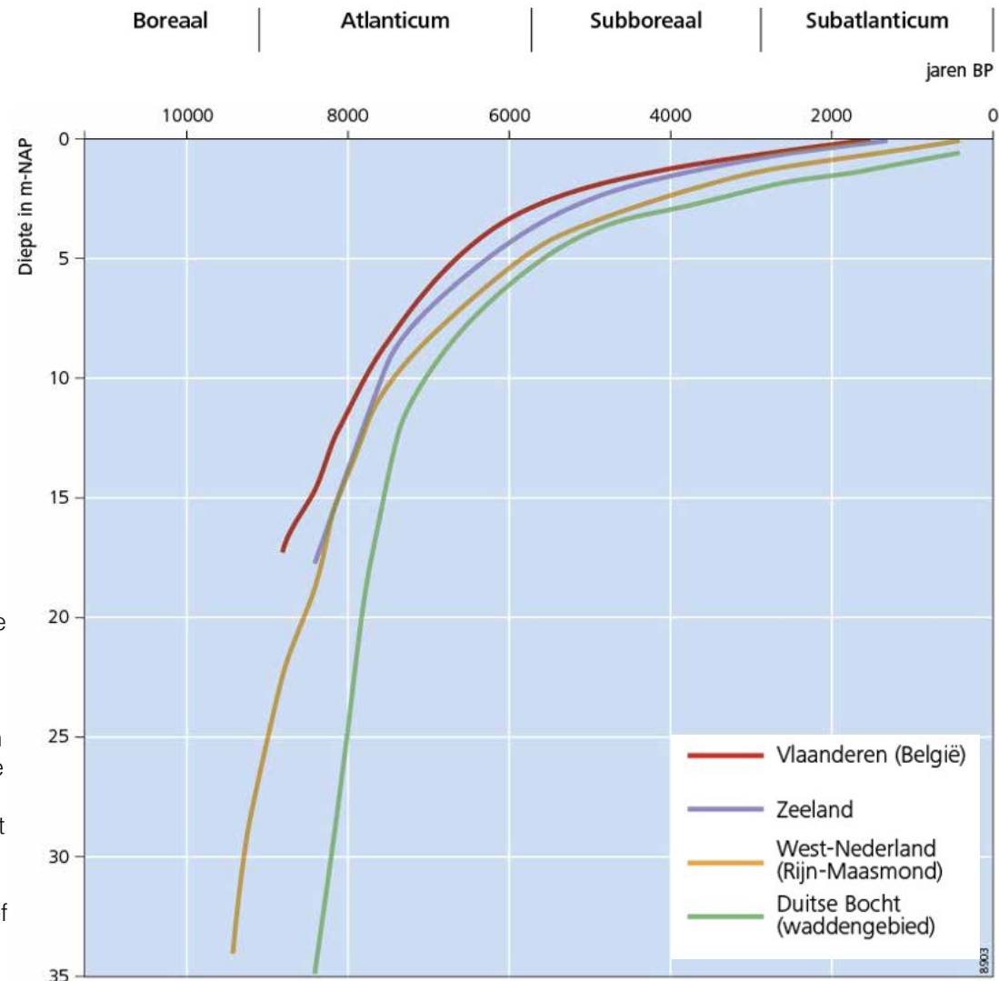
Afb.2.02 De holocene zeespiegelstijgingscurve die voor vier verschillende gebieden in Duitsland, Nederland en België is gereconstrueerd.
