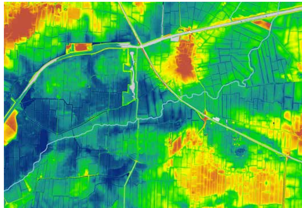
Afb.7.04 In het blauw de laaggelegen gronden, groen zijn wat hogere gronden. Direct langs de Ryd ligt een groene strook. Hier is langs het veenriviertje klei afgezet en dus is het landschap hier hoger dan in de omgeving.
