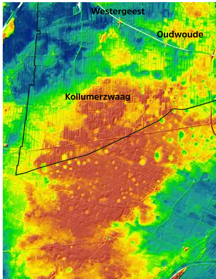
Afb.1.06 Op de hoogtekarte van Nederland is het keileemplateau met de keileemeilanden (rood/oranje/geel) en de pingoruïnes (gele en groene rondvormige laagten) zichtbaar. Voor uitleg pingoruïnes, zie Afb.1.09.
