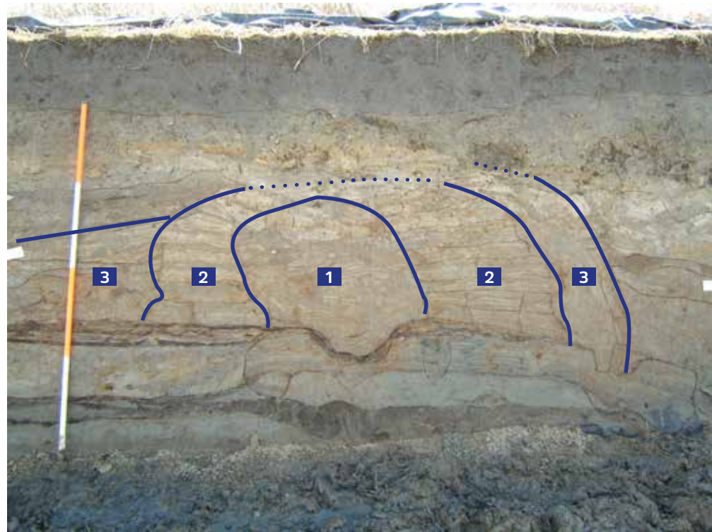
Afb.3.21 Opgeworpen dijk bij terp van Anjum, met (1) een gestort plaggenpakket als kern van de dijk. Tegen (2) de buitenzijden zijn zware, liggende plaggen gestapeld. Vervolgens zijn er (3) nogmaals plaggen gestort en liggend gestapeld aan de buitenzijden van de dijk. De zuidzijde van de dijk zal oorspronkelijk een hoek van 60 graden hebben gekend om zo, met de aanwezige begroeiing, de dijk tegen erosie te beschermen. Het bovenste deel van de dijk is vergraven (gestippeld).
