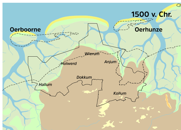
Afb.2.05 Noardeast-Fryslân en wijde omgeving op de paleogeografische reconstructiekaarten van Vos vanaf 9000 v. Chr. tot 1500 v. Chr. Via paleogeografische kaarten wordt op hoofdlijnen inzichtelijk gemaakt hoe de verdeling tussen land, zee en rivieren zich in het verre verleden heeft ontwikkeld.
