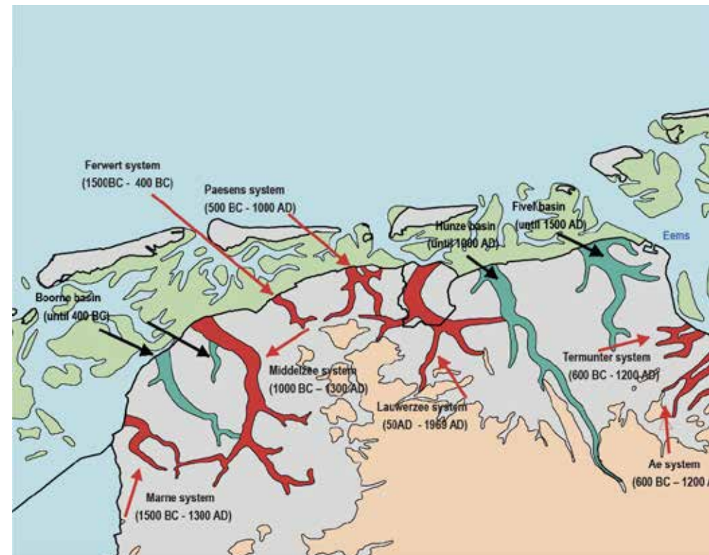
Afb.3.03 Kaart met daarop de diverse getijdengeulen die actief zijn geweest langs de Waddenkust (naar Vos, 2015).
