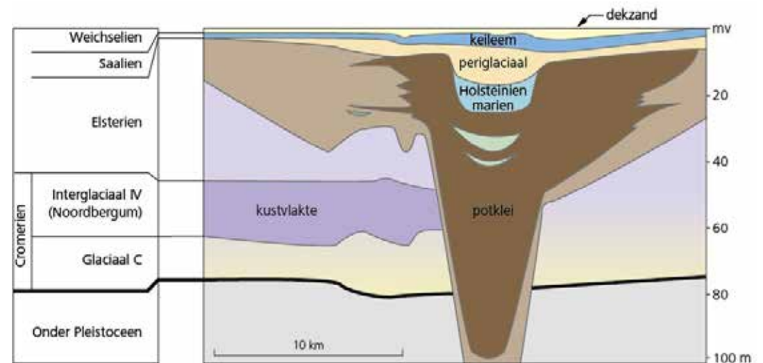
Afb.1.04 Opvulling van een tunneldal met smeltwaterzanden (lichtbruin) en potklei. Helemaal bovenin de afbeelding zijn de grondlagen aangegeven met keileem en dekzand. Dit zijn grondlagen die gevormd zijn tijdens de Saale-ijstijd (keileem) en de Weichsel-ijstijd (dekzand).
