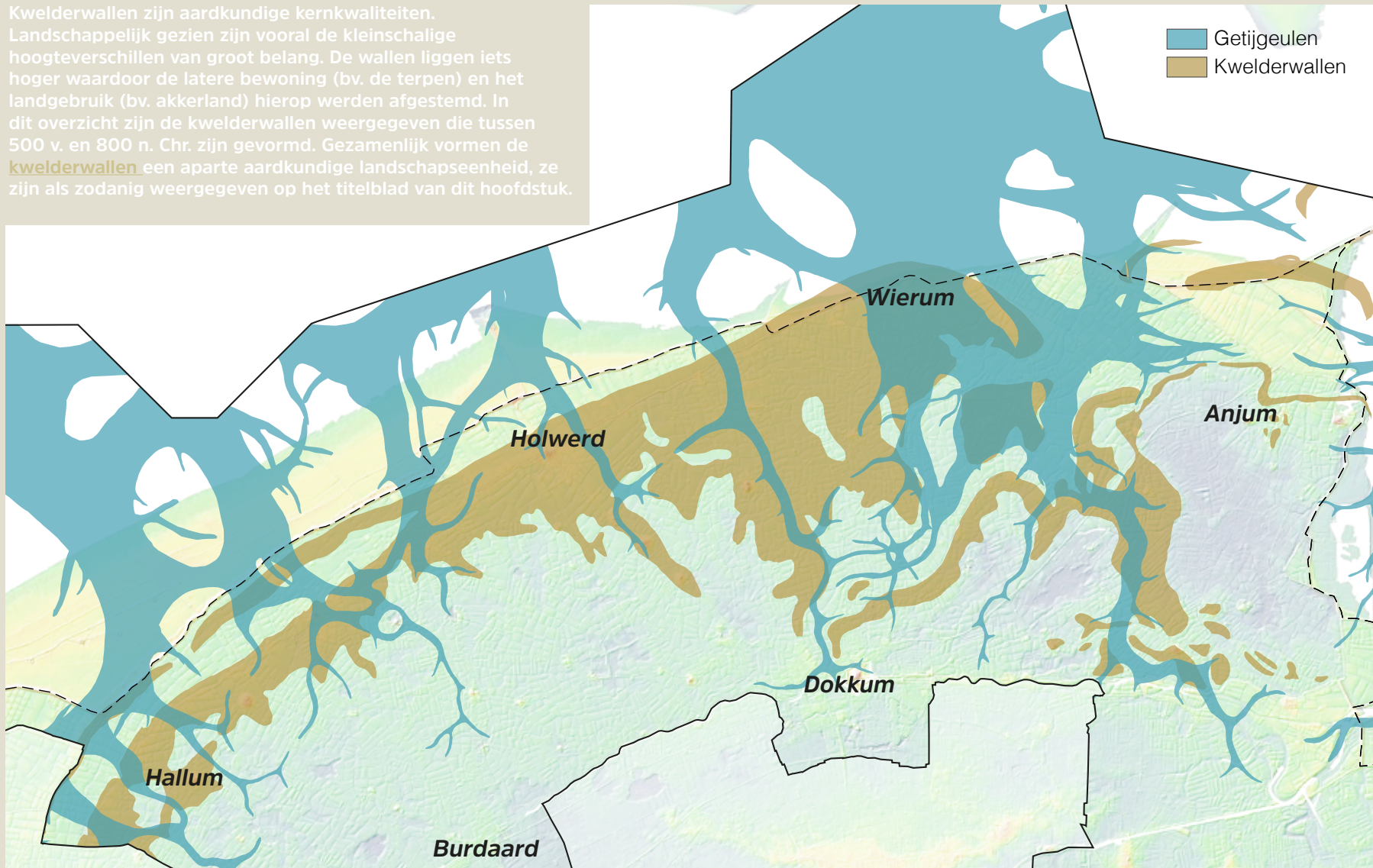
Afb.2.12 De kwelderwallen (bruin) in Noardeast-Fryslân die zijn gevormd tussen 500 v. Chr. en 800 n. Chr. (naar Vos, 2013) worden als een aardkundige kernkwaliteit beschouwd en zijn als zodanig weergegeven op de kaart met als achtergrond het hoogtebestand. Het zijn waardevolle structuren gebleken voor de bewoning en het landgebruik. Ook de getijdengeulen (500 v. Chr. – 800 n. Chr.) staan op deze kaart aangegeven (blauw).
