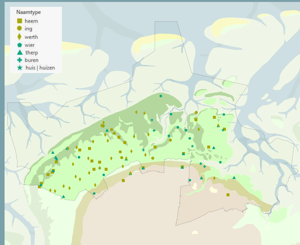
Afb.3.13 De terpnamen in Friesland weergegeven op naamtype. Opvallend is dat de jongere naamtypen (groen) zich concentreren langs het dichtgeslibde noordelijke deel van het Peazens-systeem. Ook langs het latere Dokkumer Grutdijp en in de veenrandzone liggen overwegend jongere naamtypen.
