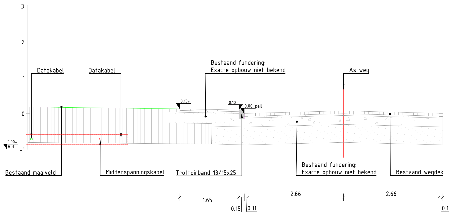
Principe dwarsprofiel Bestaande situatie 1:50
