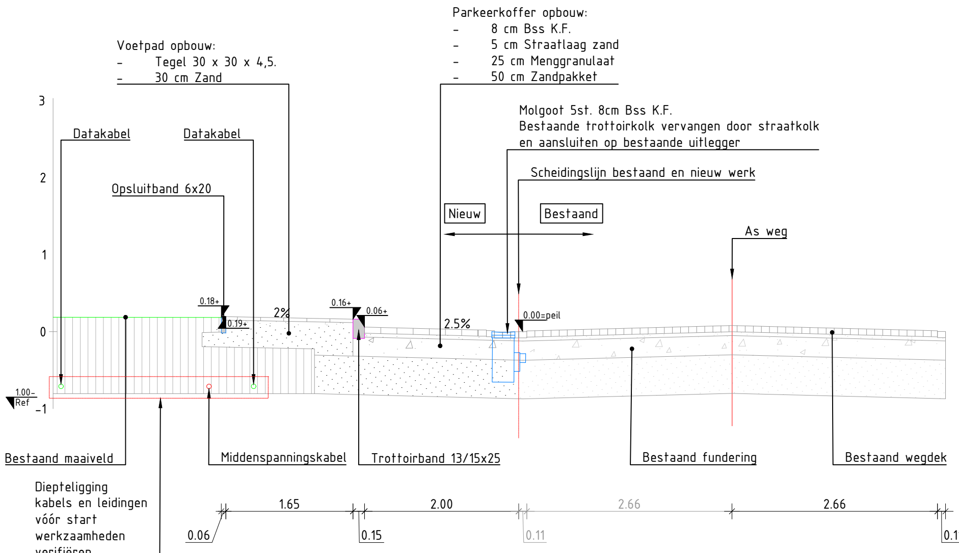
Principe dwarsprofiel Nieuwe situatie 1:50
