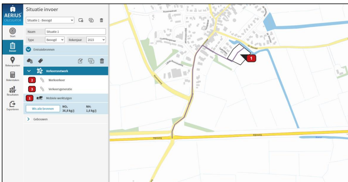
Afbeelding 3 - AERIUS-model
