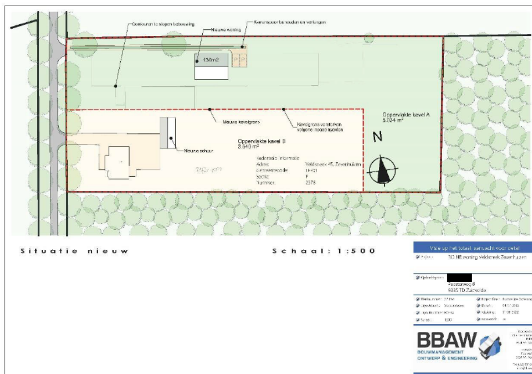
Figuur 1 stedebouwkundig ontwerp (rood omlijnd) bron: BBAW
