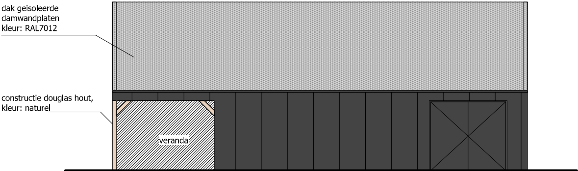
Zuidgevel
