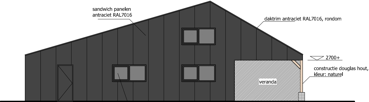
Oostgevel
