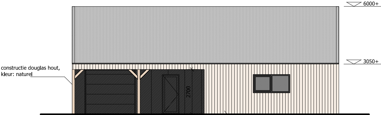
Noordgevel
