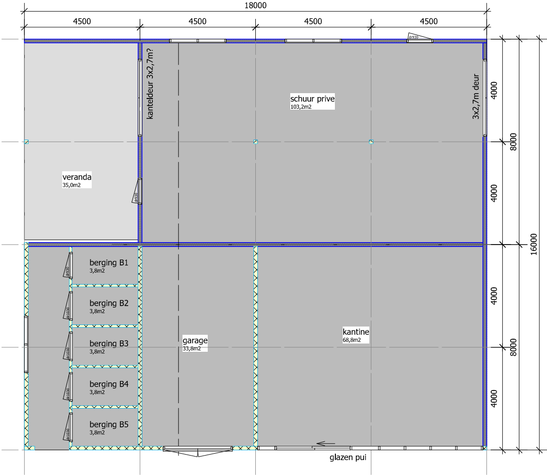
Plattegrond
