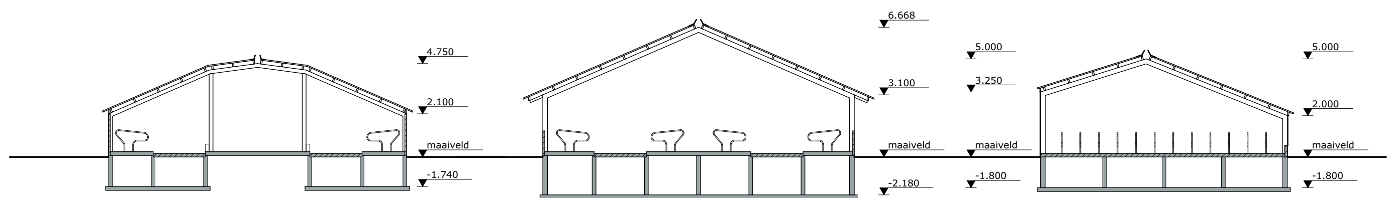
Doorsnede D-D
