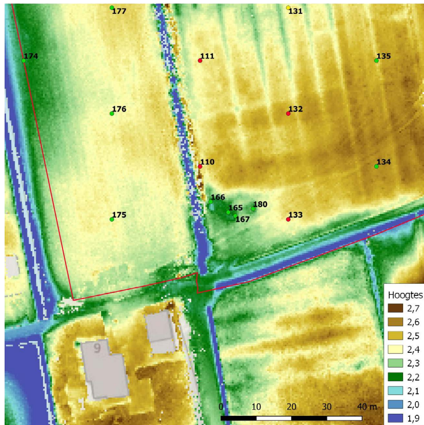
Figuur 4: Marum, Kruisweg 43: boringen in het zuidelijke deel van het plangebied met een hoogtekartaal als achtergrond. Ter plaatse van boringen 165, 166, 167, 180 is hoogstwaarschijnlijk een dobbe gedempt. Door nazakking is het een lage plek geworden.
