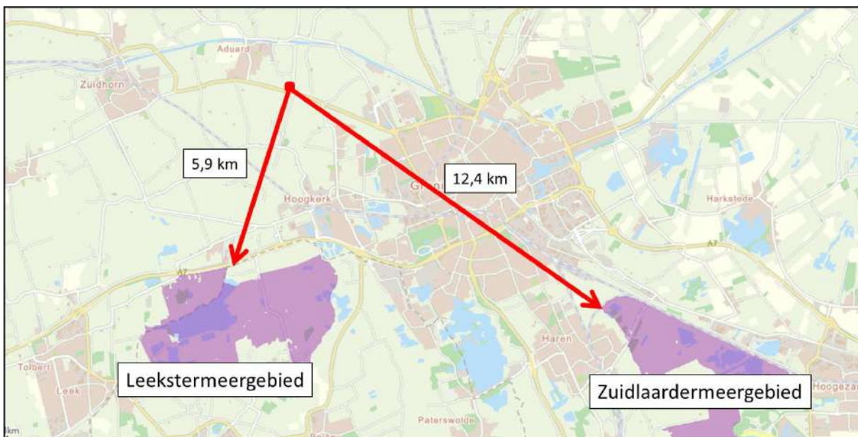
Figuur 2.9. Natura2000 (paars) gebieden in de omgeving van het plangebied (rood) (bron: Kaartenkijkdoos Provincie Fryslân).
