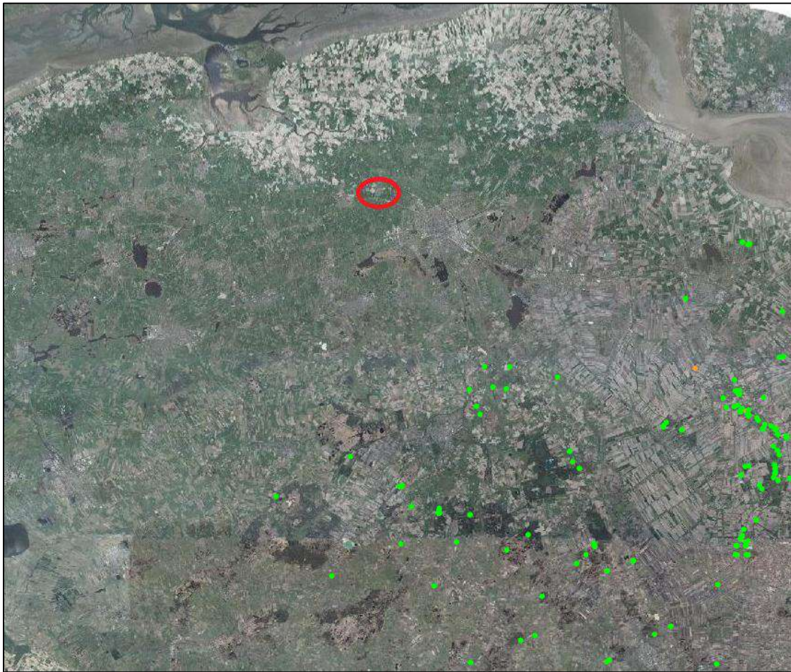
Figuur 2.6. In de directe omgeving van het plangebied (rood omlijnd) zijn geen waarnemingen van grote bosmuis (groene stippen) bekend (bron: NDFF).
