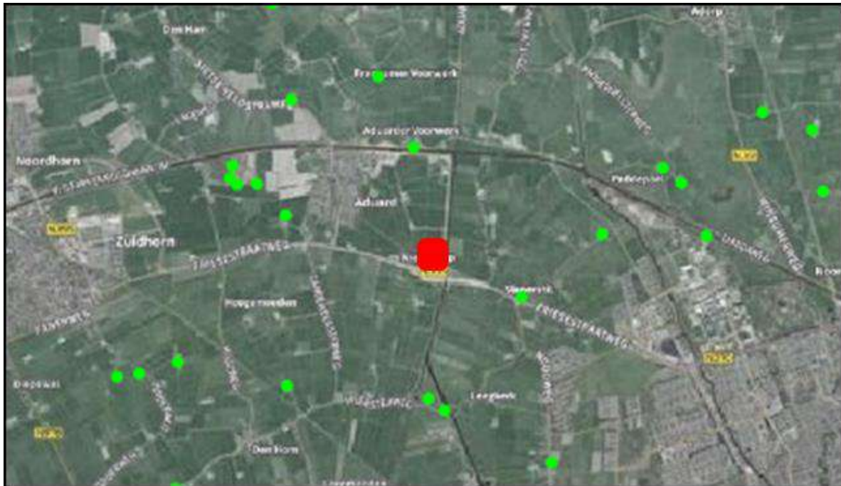
Figuur 2.6. Waarnemingen van waterspitsmuis (groen gemarkeerd) in de omgeving van het plangebied (rood)(Bron: NDFP).
