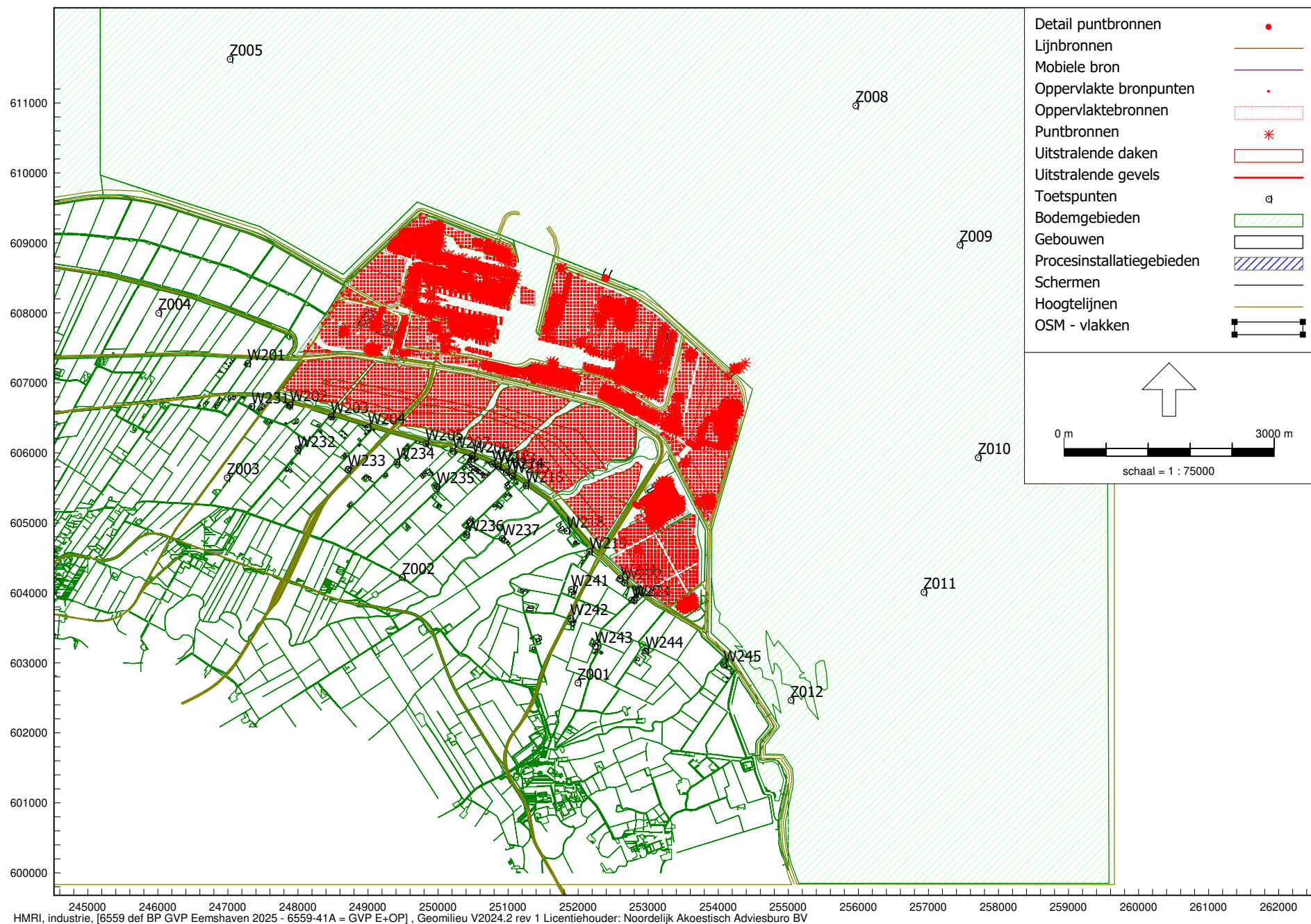
Overzicht geluidverdeelmodel (bodembgebieden gearceerd)
