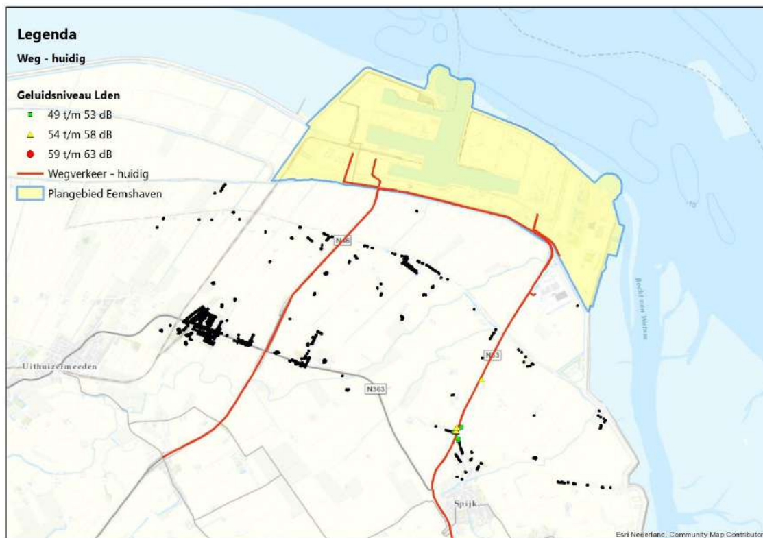
Abbeelding 6.4 Resultaten wegverkeer in de huidige situatie
