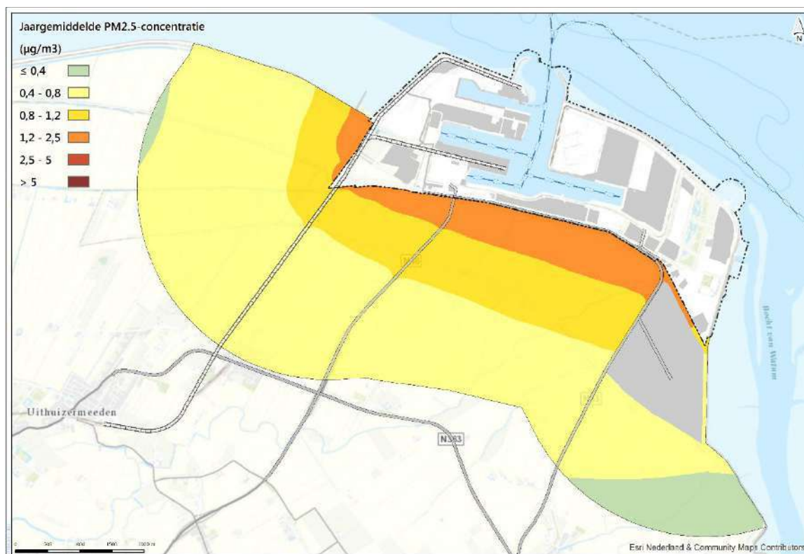
Afbeelding 7.12 Toename van de jaargemiddelde PM2.5-concentratie in 2030: plansituatie (maximaal scenario) - referentiesituatie
