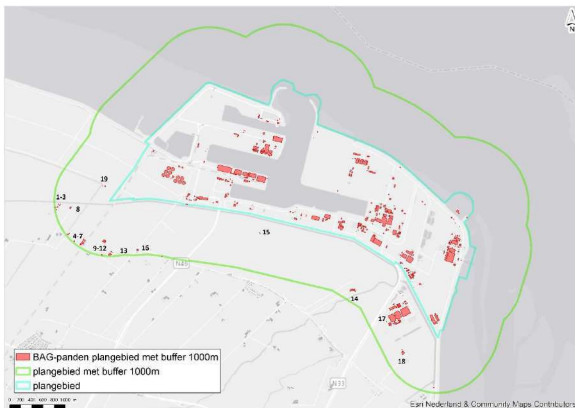
Afbeelding 9.7 Maximale 10^{-6} -plaatsgebonden risicocontour
