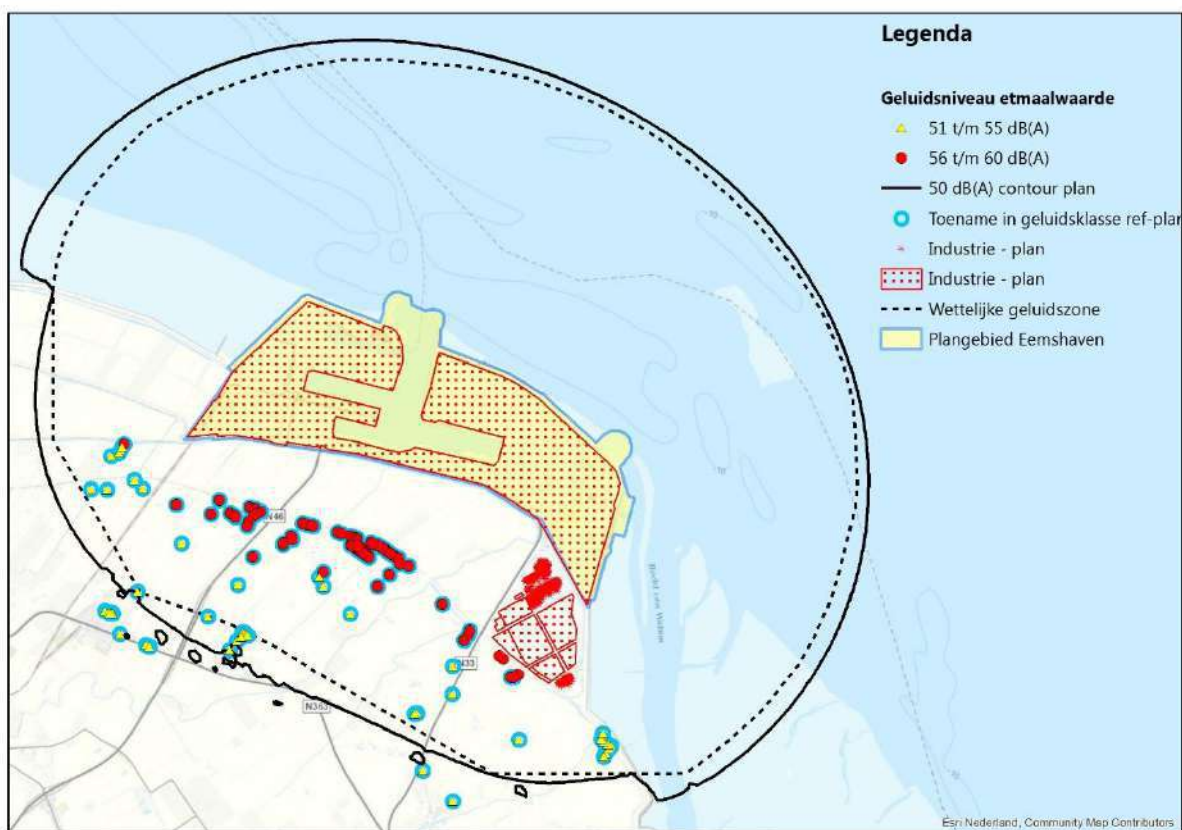
Afbeelding 6.10 Industrielawaai bij een maximaal scenario (gevoeligheidsanalyse)
