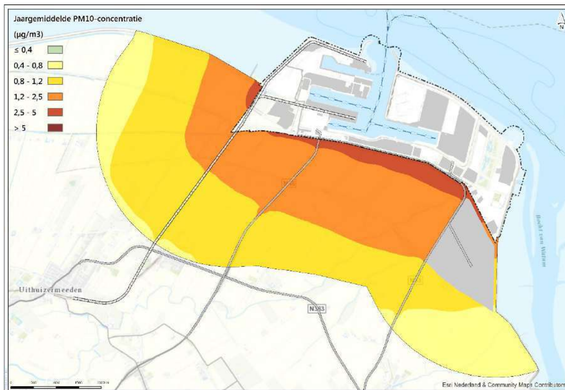
Afbeelding 7.11 Toename van de jaargemiddelde PM10-concentratie in 2030: plansituatie (maximaal scenario) - referentiesituatie
