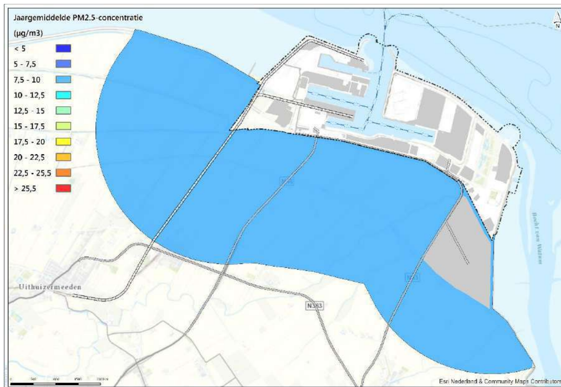
Afbeelding 7.9 Jaargemiddelde PM2.5-concentratie - Plansituatie (maximaal scenario) - 2030
