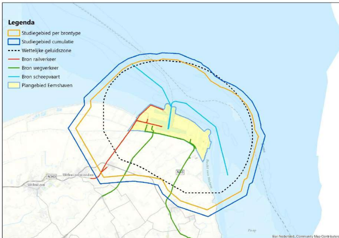
Afbeelding 6.1 Situering brontypen geluid en studiegebieden
