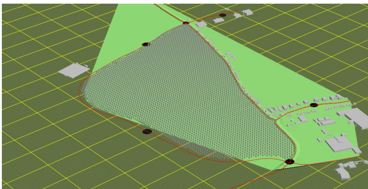
3D – wegverkeerslawaaai
