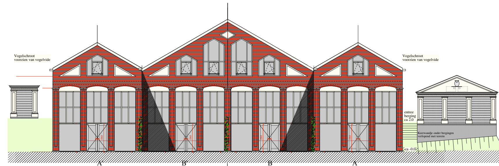
AANZICHT DIJKZIJDE
