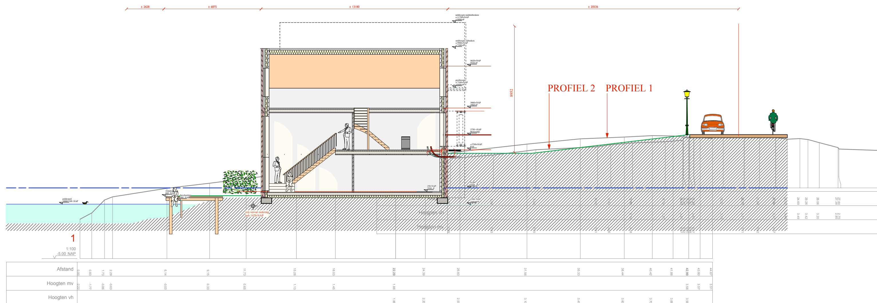
DOORSNEDE, DIJKPROFIEL
