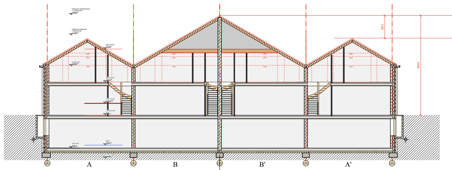
DOORSNEDE
