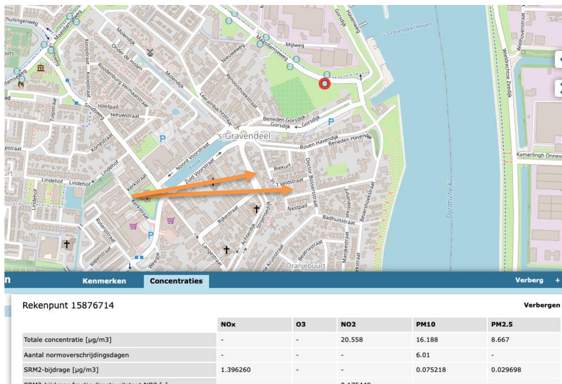
Figuur 4.8: NSL-monitoringstool
