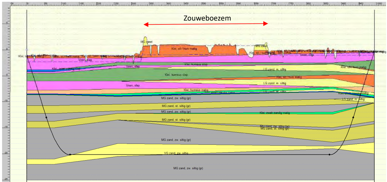
Figuur 2.3: lang profiel HDD onder Natura 2000-gebied Zouweboezem
