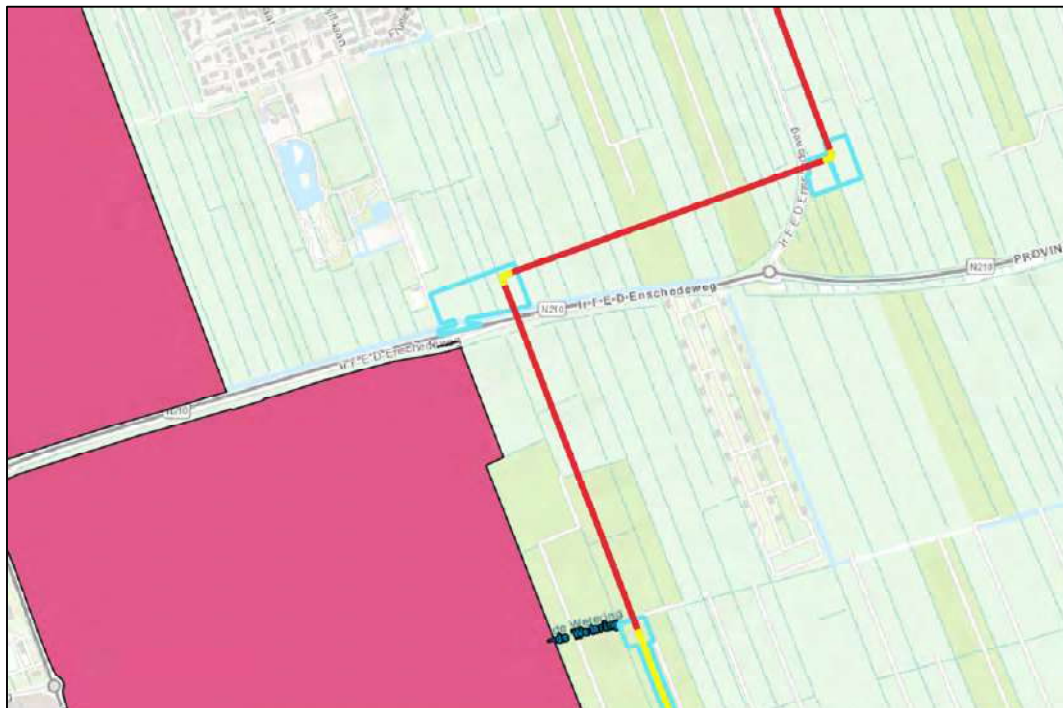
Figuur 4.43. Ligging van het HTL tracé (rood = HDD, geel = open ontgravingen) en de werkstroken (blauw) ten opzichte van de weidevogelkerngebieden (roze). Het HTL loopt nabij de N210 langs een weidevogelkerngebied (bron achtergrond: Esri).
