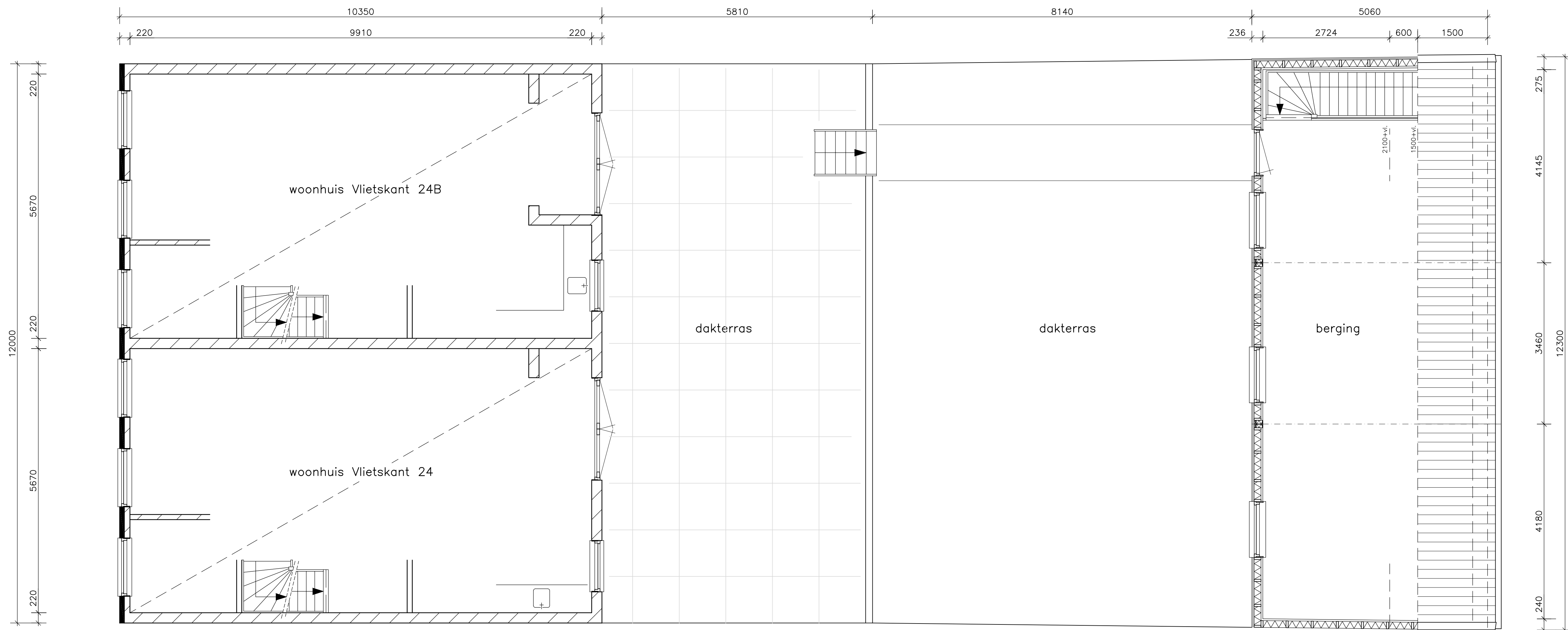
1e verdieping
