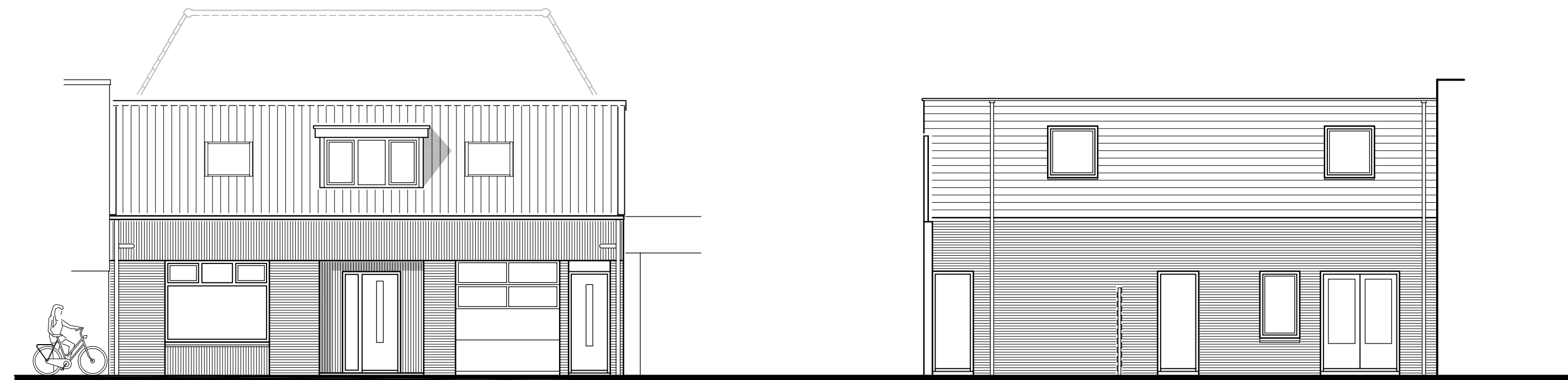
vooraanzicht Oostwal
