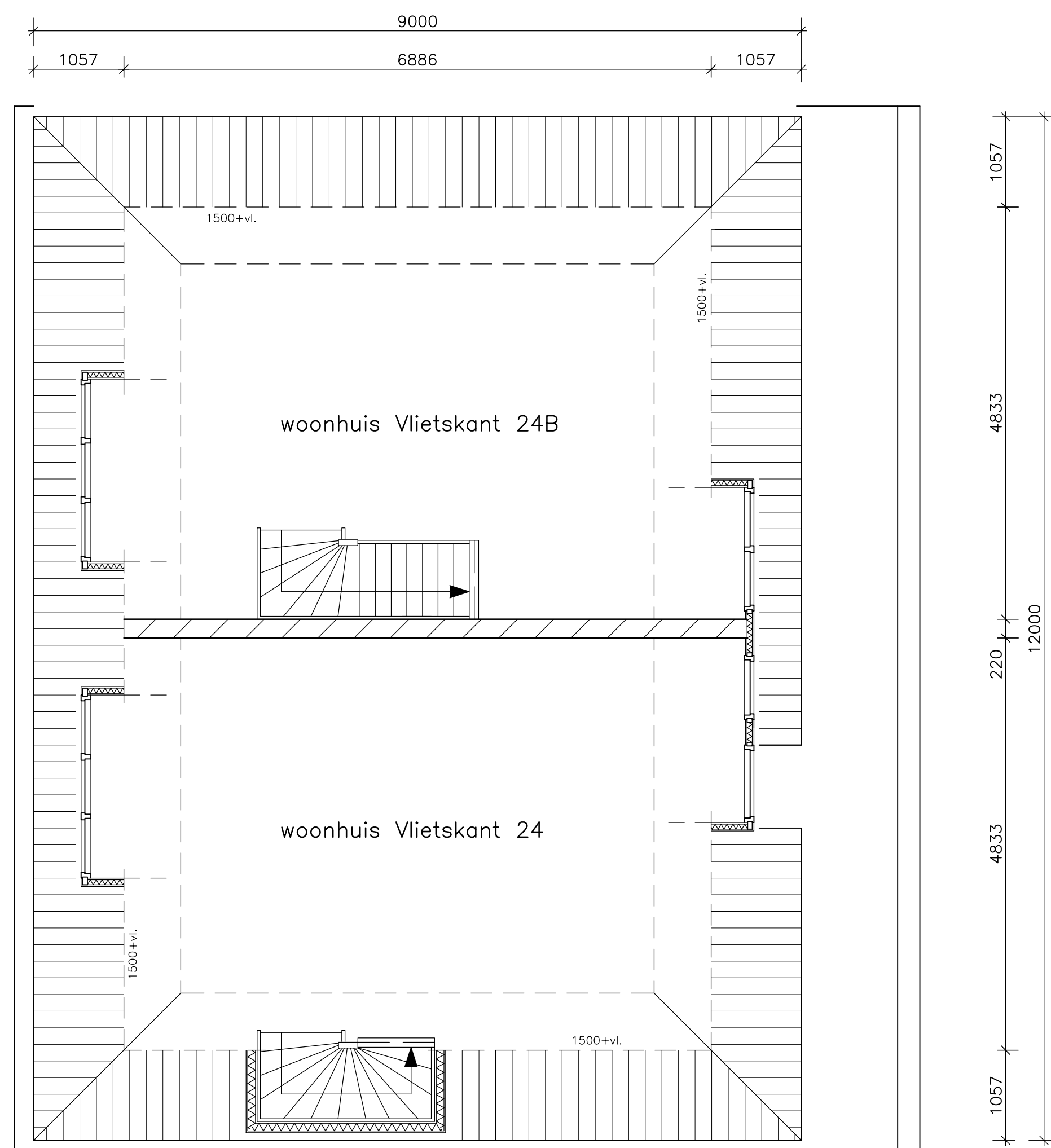
2e verdieping
