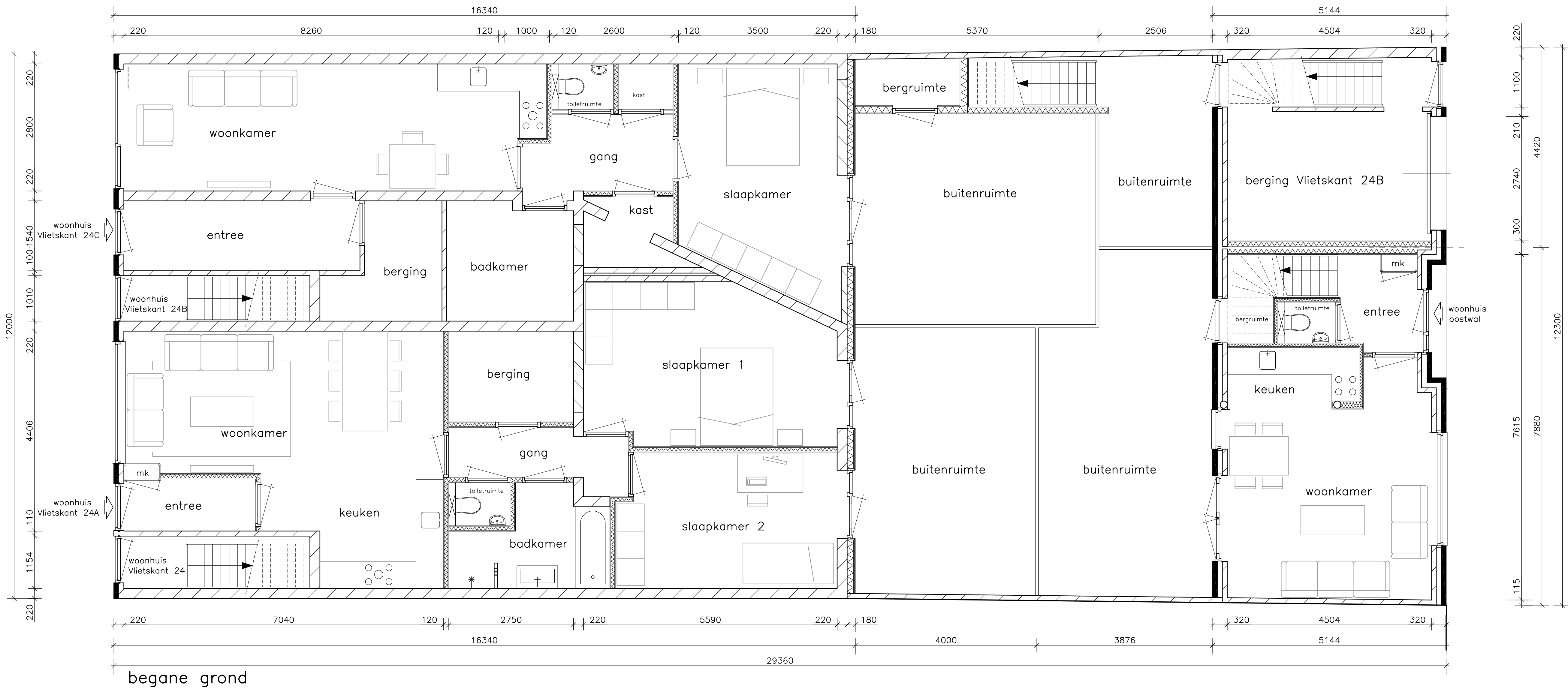
begane grond
