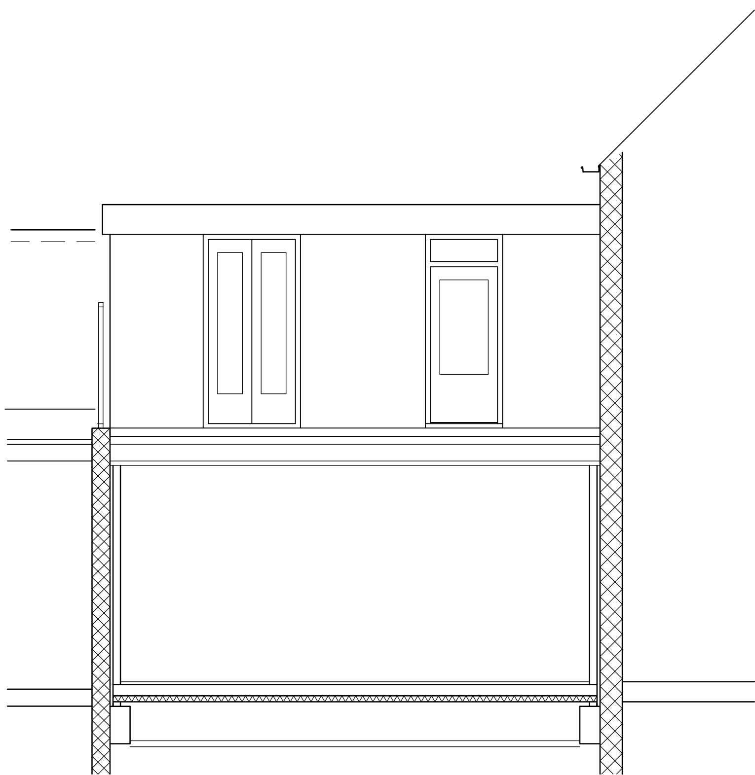
dwarsdoorsnede D en aanzicht gevel woning Oostwal
