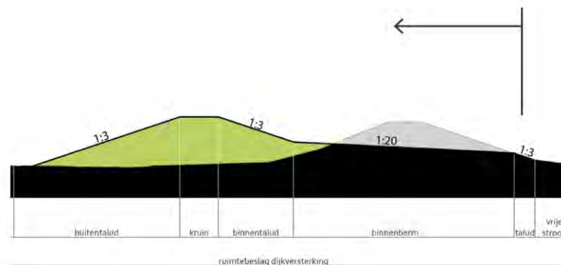
Schematisch dwarsprofiel dijkversterking grond buitenwaarts. Bron: Graaf Reinald Alliantie, 24 april 2018.
