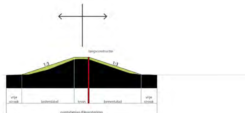
Schematisch dwarsprofiel dijkversterking langsconstructie. Bron: Graaf Reinald Alliantie, 24 april 2018.
