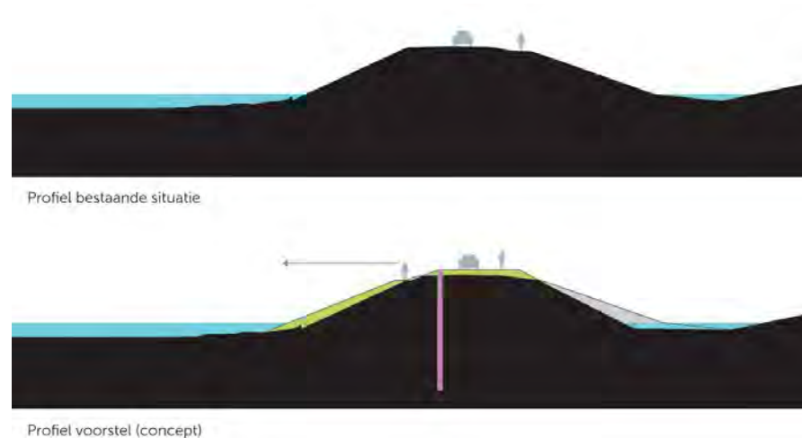
Schetsontwerp locatie Vesting Gorinchem. Bron: Veenenbos en Bosch landschapsarchitecten, 12 juli 2018.
