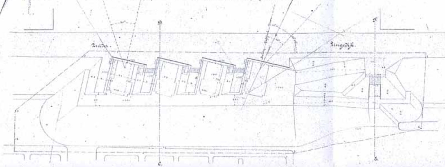
Fig 2. Plan van het emplacement in oorlogstijd. 1:200.
