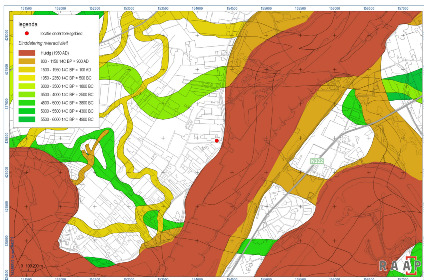
Figuur 5.1 Meandergordels in de omgeving van Varik, uit Cohen e.a. 2012.
