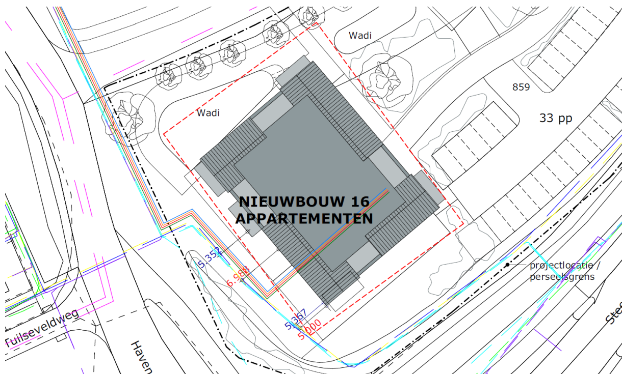
Afbeelding 18: Situatietekening met leiding-/kabeltracés
