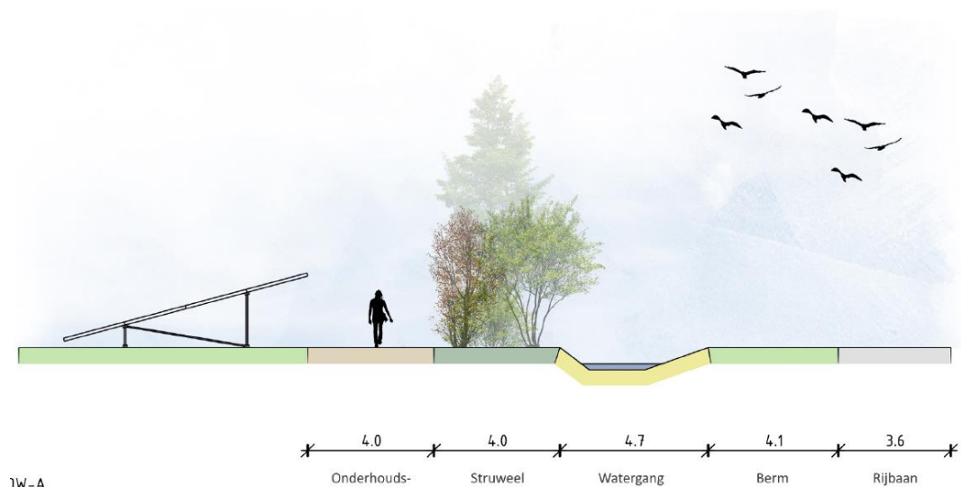
Figuur 2.4: dwarsdoorsnede vanaf de Haarweg
