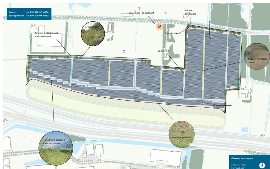
Figuur 1.2: Landschappelijk inpassingsplan (bron: Antea Group, 2020)
