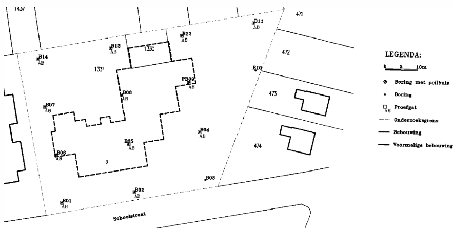
Afbeelding 3: situatietekening met boorpunten en asbestinspectiegaten (bron tekening: Verhoeven Milieutechniek B.V.)
