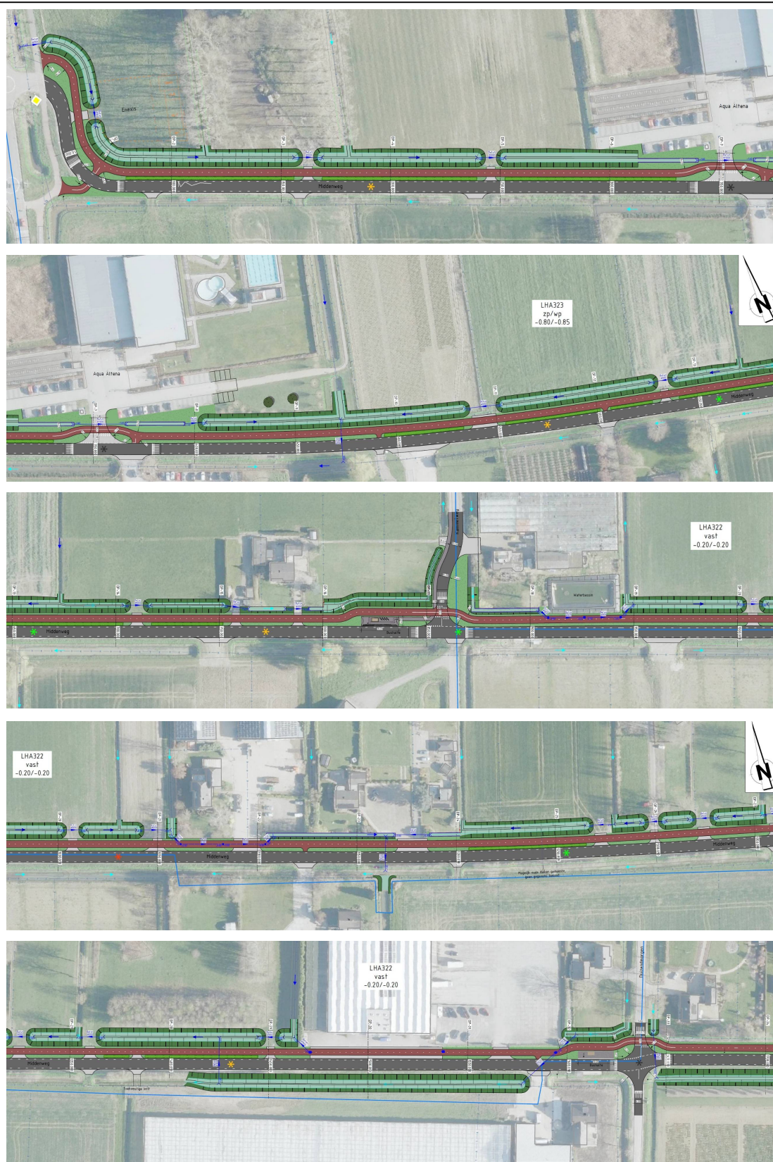
Figuur 13 – Inrichtingstekening nieuw fietspad Middenweg Andel - Veen (bron: Geo Infra B.V., 25 juli 2024)
