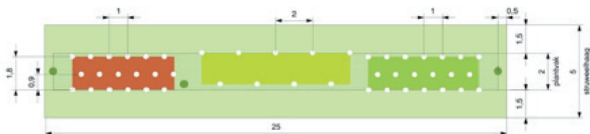
Bovenaanzicht: Aanleg
