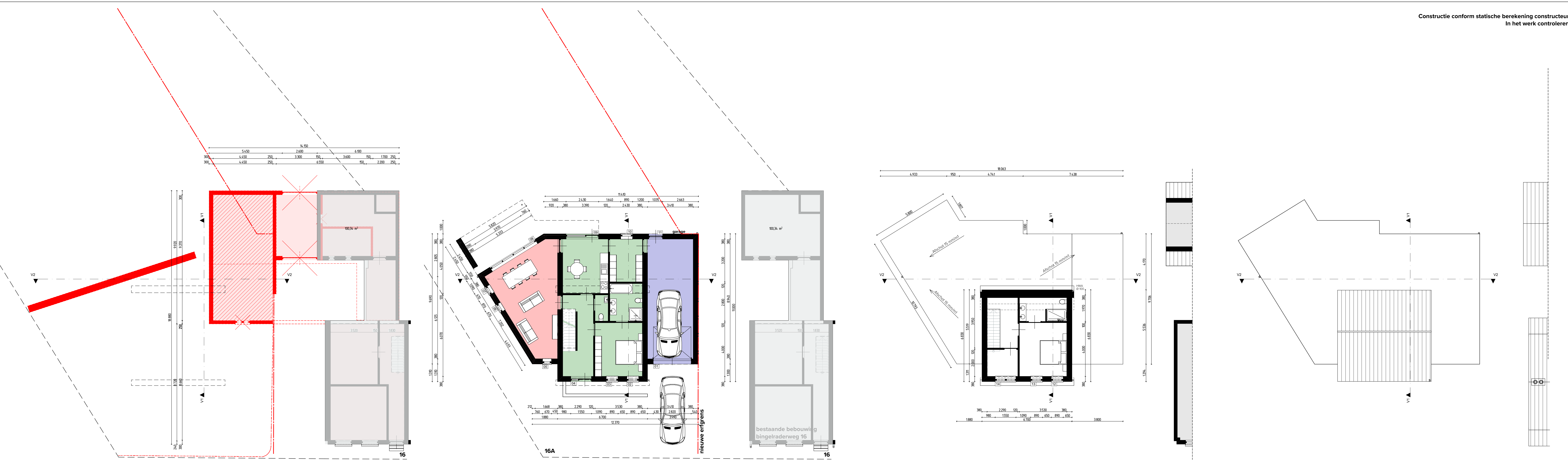
Begane grond (Sloop) Begane grond (Ontw) 1e verdieping (Ontw) dakaanzicht (Ontw)
