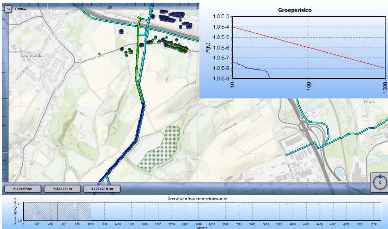
Figuur 4-14 Groepsrisico buisleiding A-534 huidige en toekomstige situatie (maatgevende kilometer)
