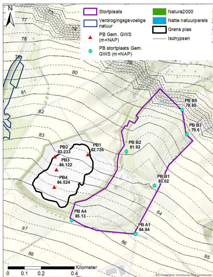
Figuur 4-3 Berekende grondwaterstand Ibrahim V22 Z (isohypsen) en gemeten gemiddelde grondwaterstanden bij de beschikbare peilbuizen, gekalibreerd
