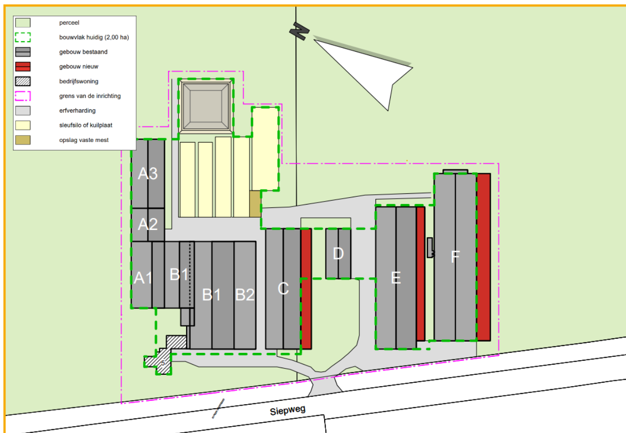
Figuur 2. Situatieschets van de gewenste situatie (Bron: Agra-Matic). Met rood is de nieuwe overdekte uitloopruimte weergegeven.
