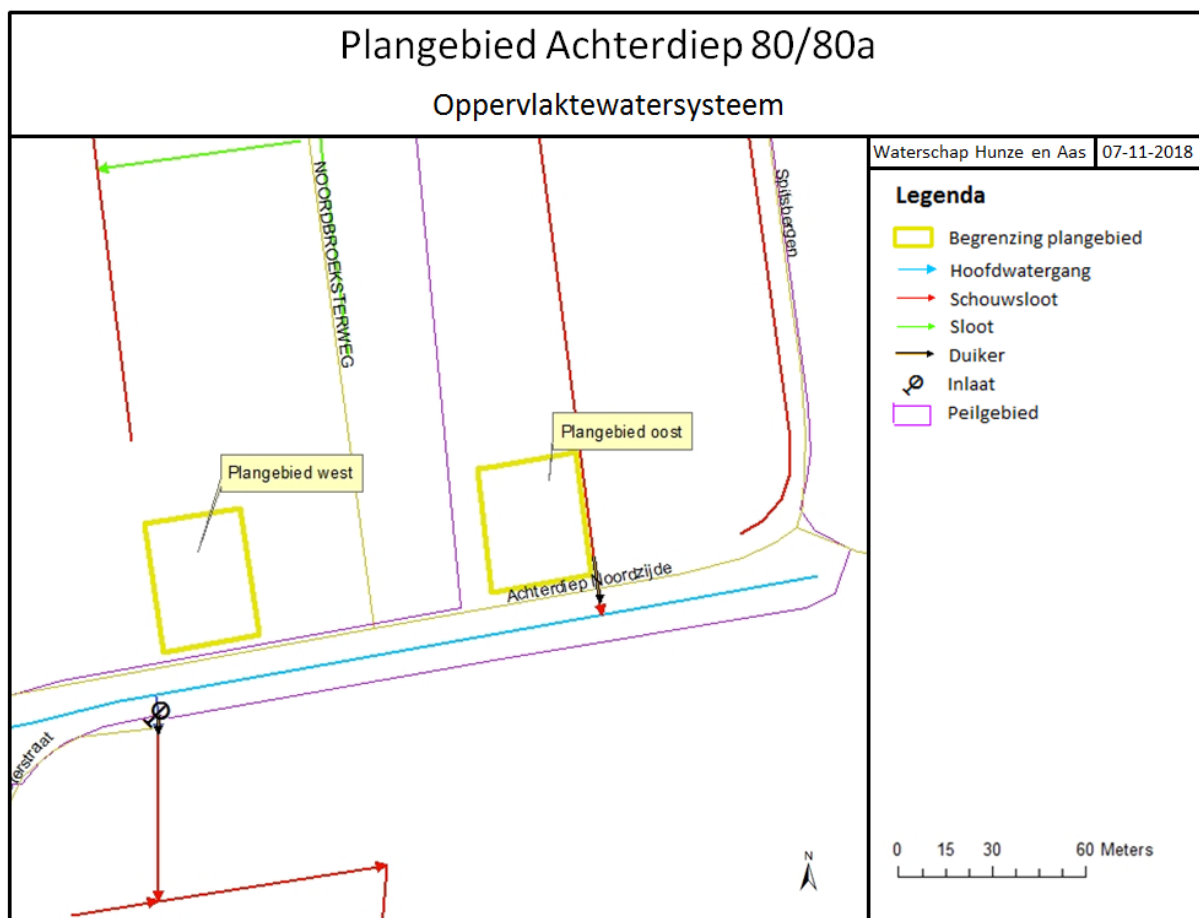
Figuur 1 Oppervlaktewatersysteem
